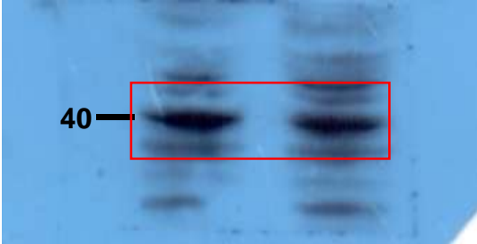
WCE: \alpha -FAM47E
