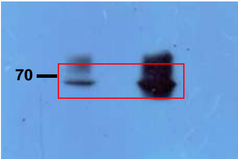
IB: \alpha -PRMT5
