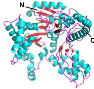
E PrmA ( E. coli )
