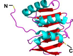
D aKMT ( Sulfolobus islandicus )
