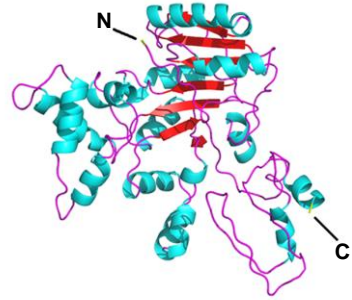
D aKMT ( Sulfolobus islandicus )
