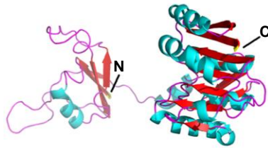
E PrmA ( E. coli )
