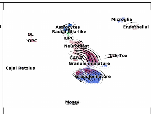
kallistobus_coll_excl
