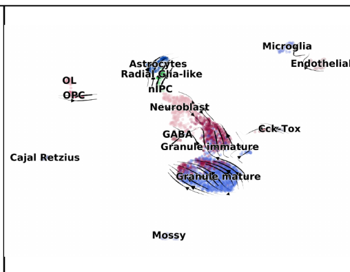
kallistobus_sep_excl
