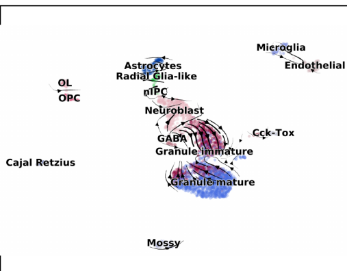
alevin_sep_gtr
