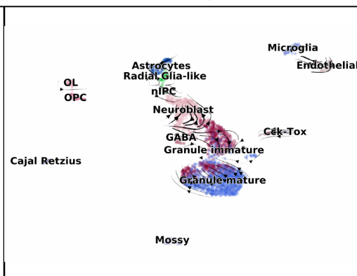
starsolo_diff
