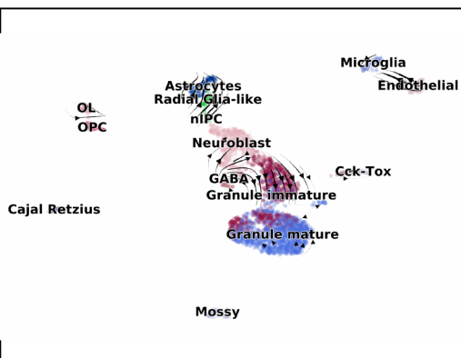
starsolo
