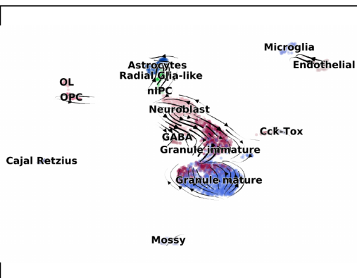
kallistobus_coll_incl
