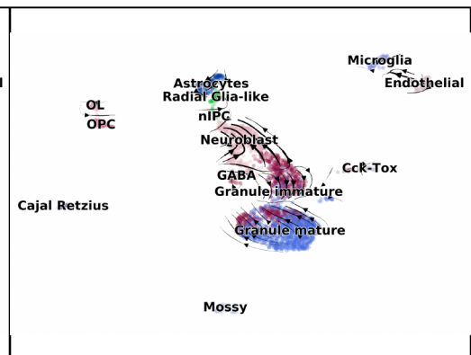
kallistobus_sep_incl
