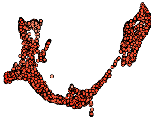
kallisto|bus_sep_excl
