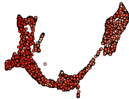
velocyto
