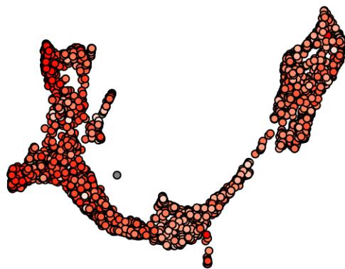
starsolo
