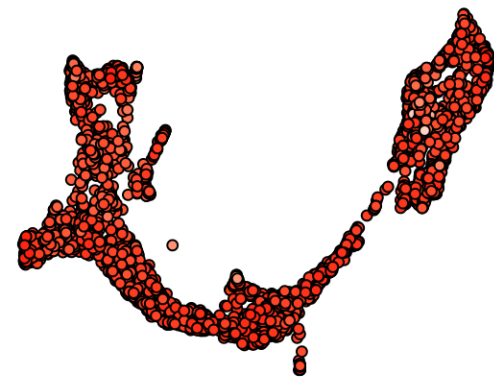
kallisto|bus_coll_excl
