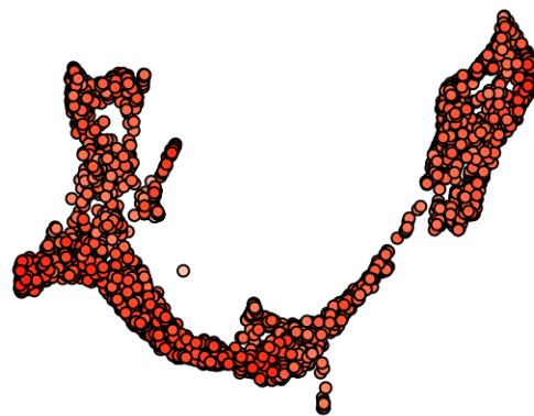
starsolo_diff
