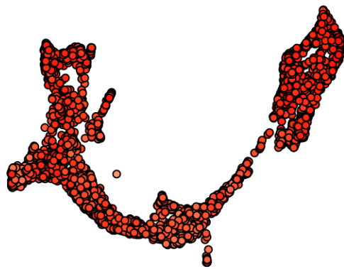
kallisto|bus_coll_incl
