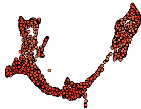
alevin_sep_gtr
