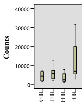
NUPR1
