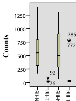
DIRAS1
