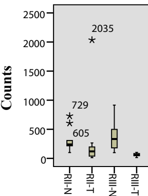
ANKRD22
