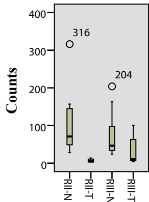
NAT2
