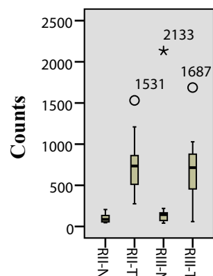
TPX2
