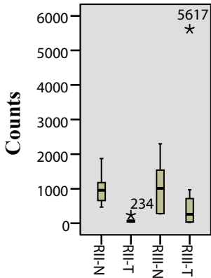
CKMT2
