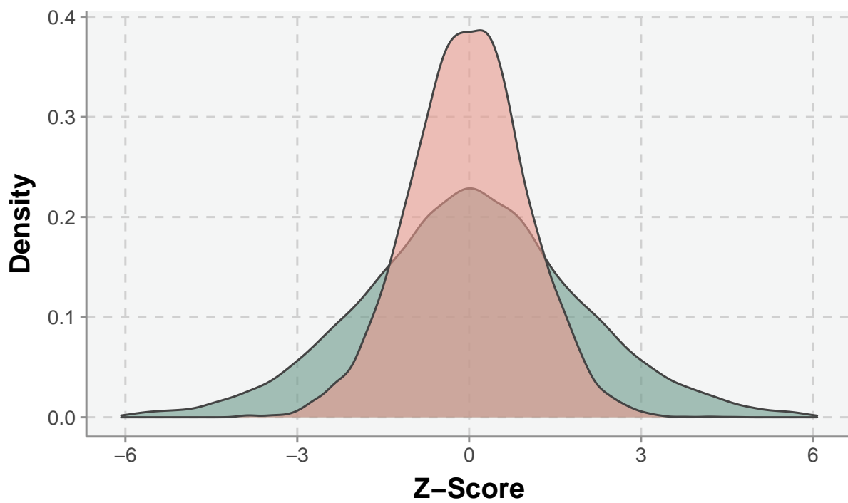
ALS Meta-Analysis
