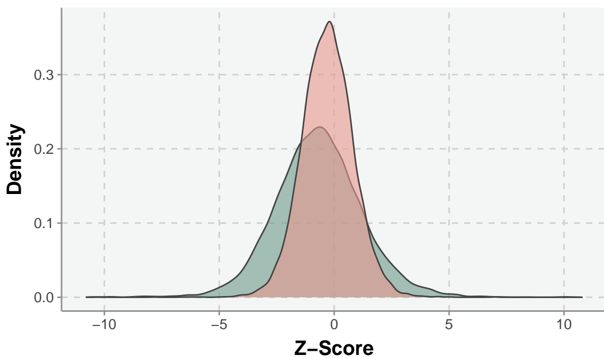
ALS Meta-Analysis
