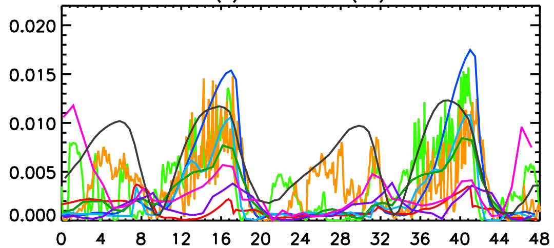
(h) Wind stress (Pa)
