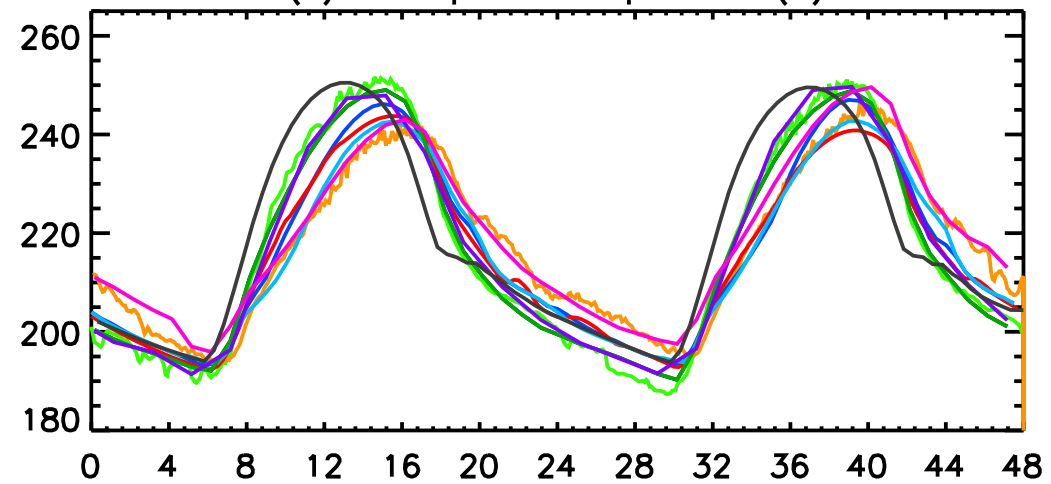
(d) Atmospheric temperature (K)
