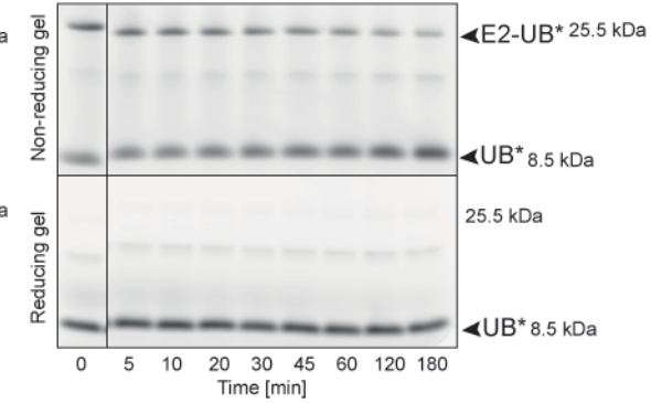
L-Serine
