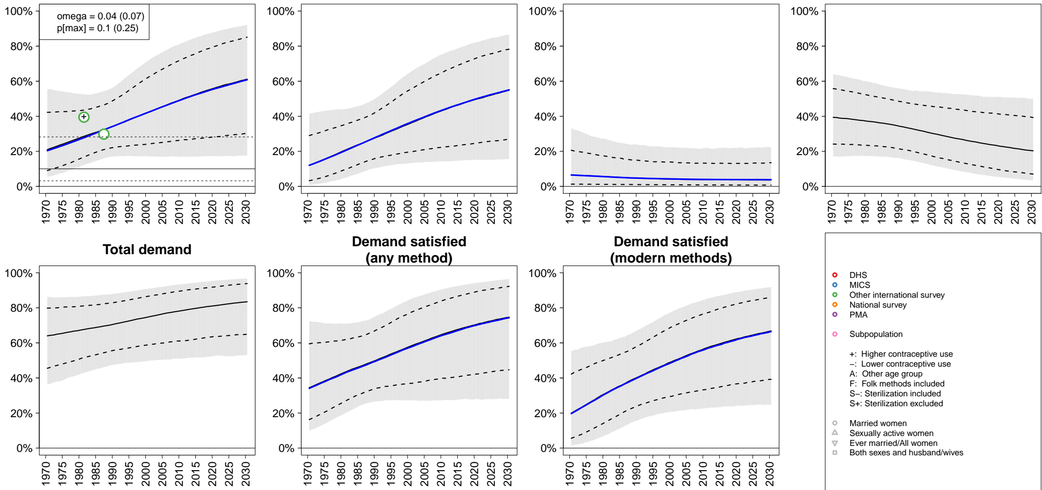
CP (any)
