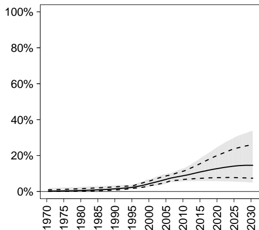
CP (modern)
