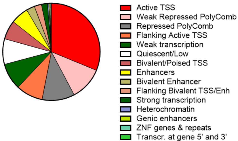
chromHMM All CpG Clusters
