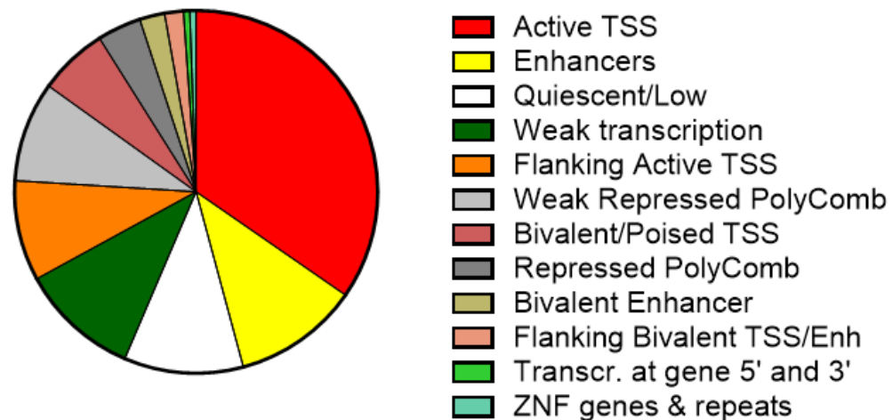
chromHMM FDR Clusters
