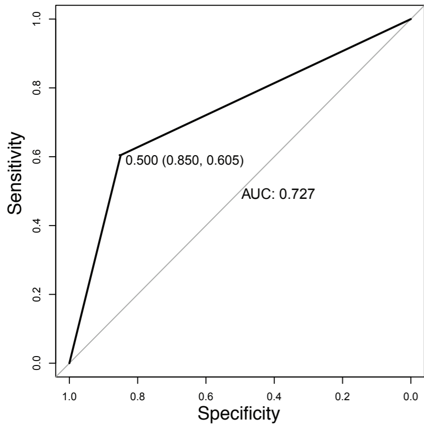
BNP
