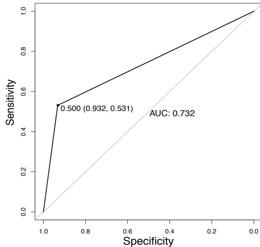
hs-TNI
