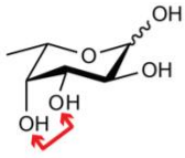
L-Fucopyranose
