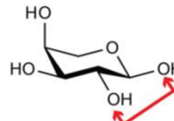
\alpha -L-Arabinopyranose
