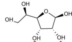
\alpha/\beta -D-Allofuranose
