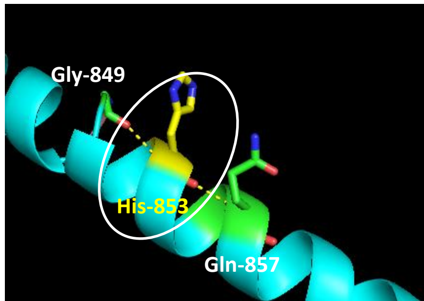
MYO7A p.Arg853His
