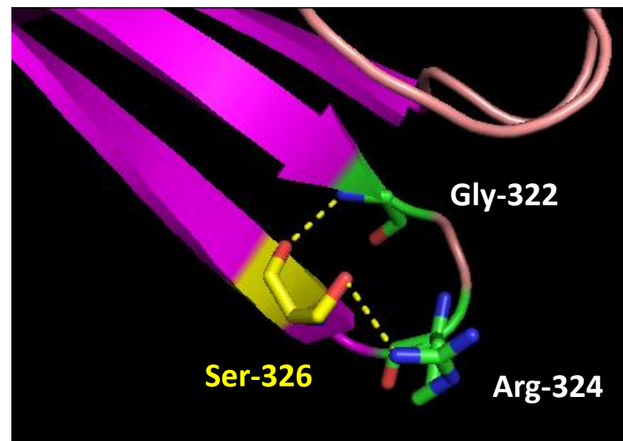
LOXHD1 p.Asn326Ser
