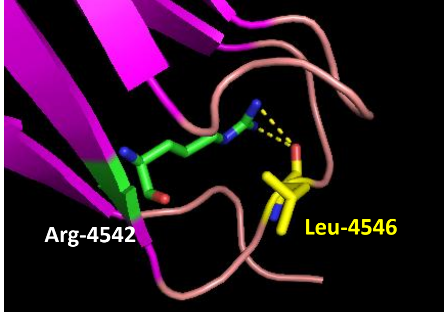
ADGRV1 p.Leu4546
