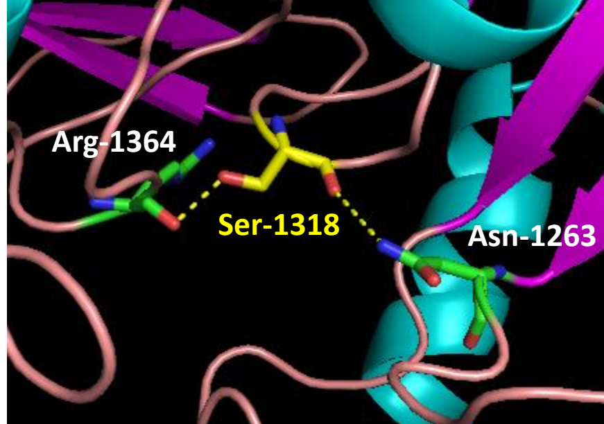
MYO15A p.Gly1318Ser
