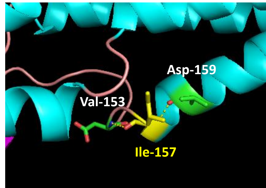
GJB2 p.Met157Ile
