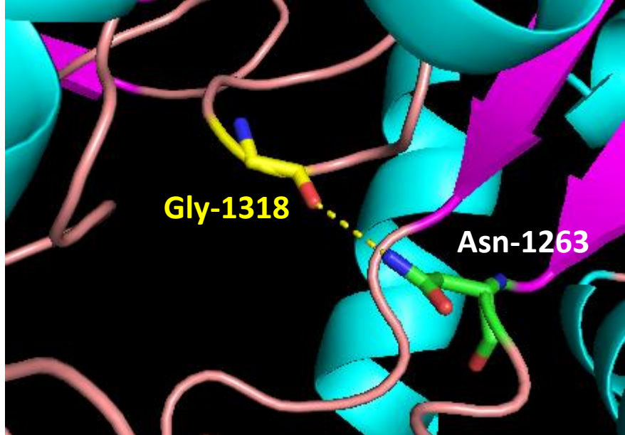
MYO15A p.Gly1318
