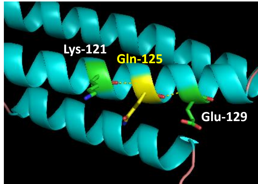
TMC1 p.Lys125Gln
