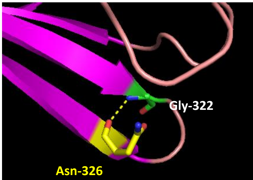
LOXHD1 p.Asn326
