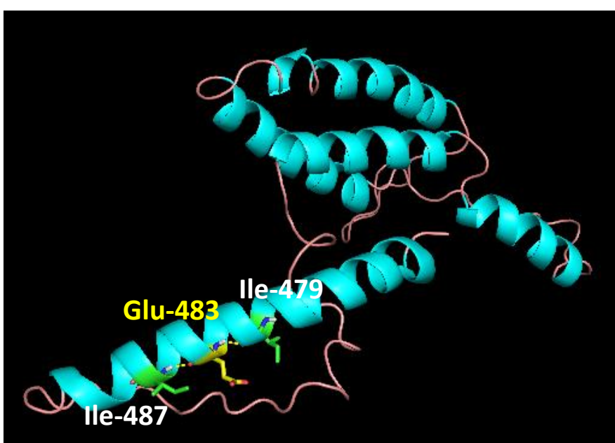
TMC1 p.Glu483
