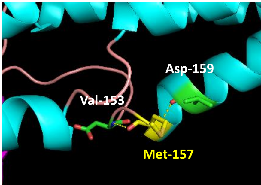
GJB2 p.Met157
