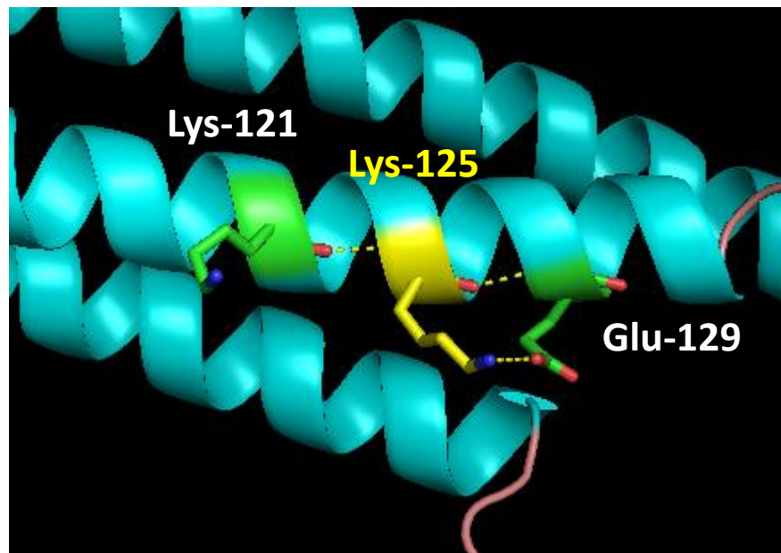
TMC1 p.Lys125
