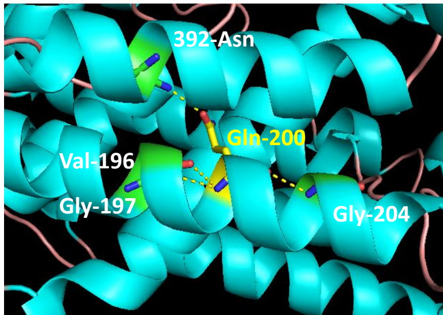
SLC26A4 p.Gln200
