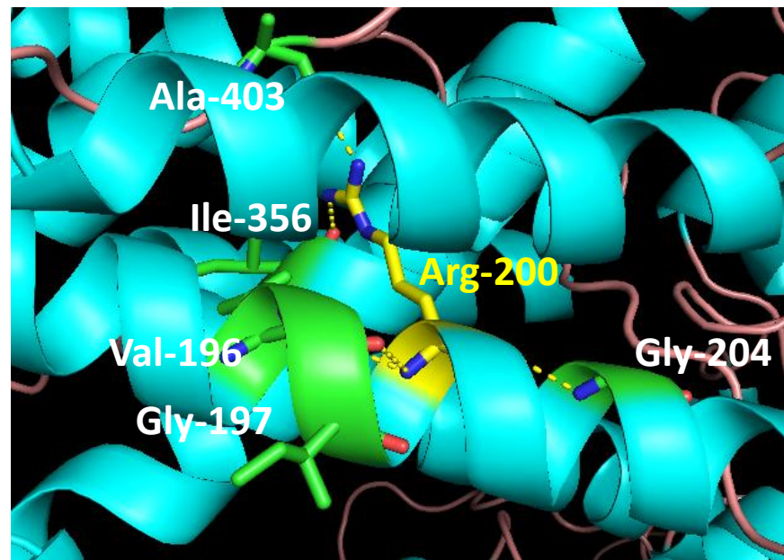
SLC26A4 p.Gln200Arg
