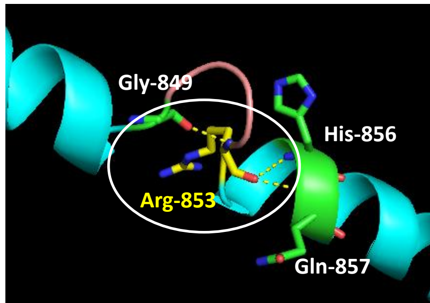
MYO7A p.Arg853
