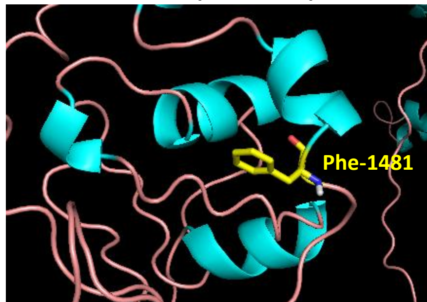
TMC1 p.Glu483Asp
