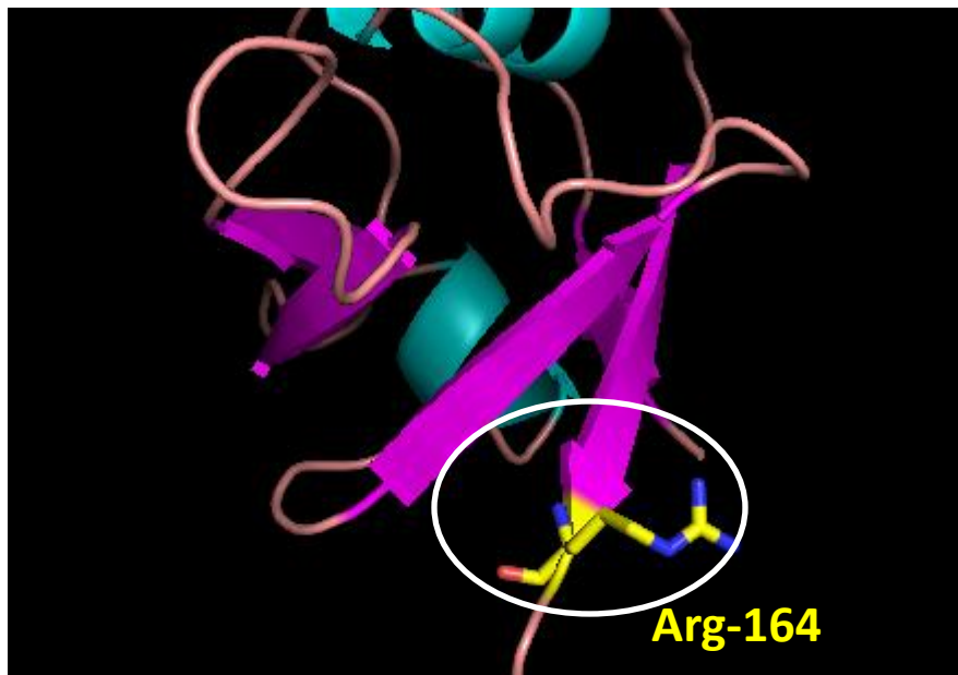
PDZD7 p.Arg164
