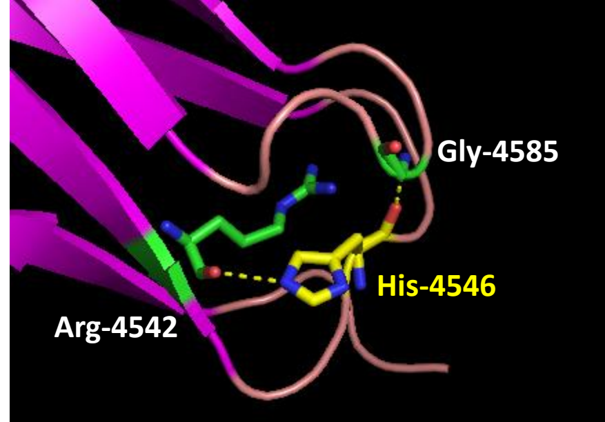
ADGRV1 p.Leu4546His
