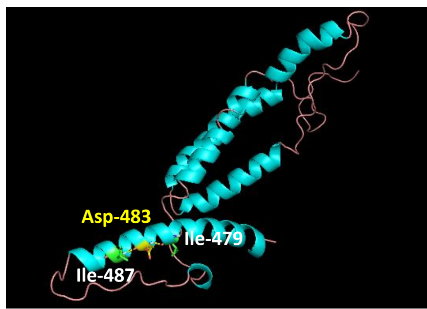
TMC1 p.Glu483Asp
