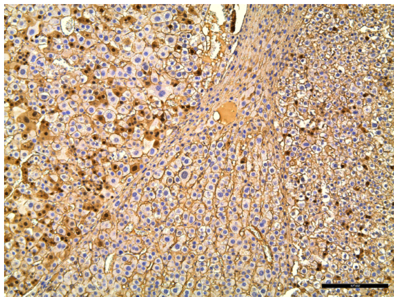
c-Met/sgApc
