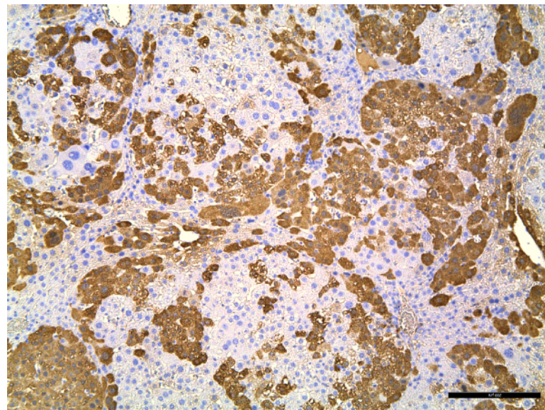
GLUL (100X)
