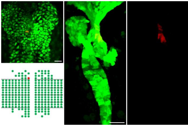
L-A-c1r4 (n=5)
