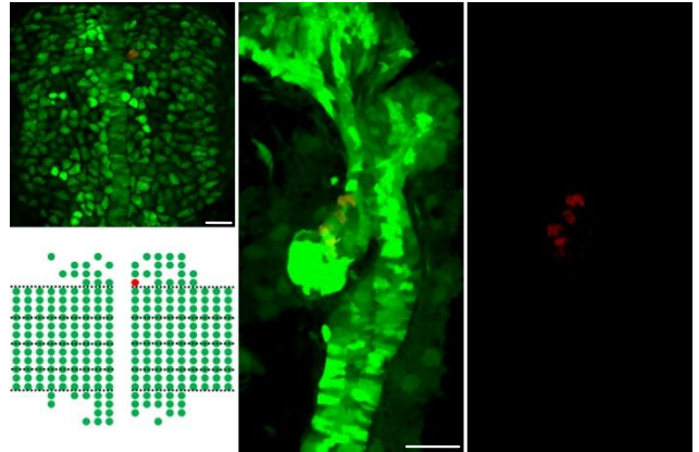
R-A-c1r4 (n=5)
