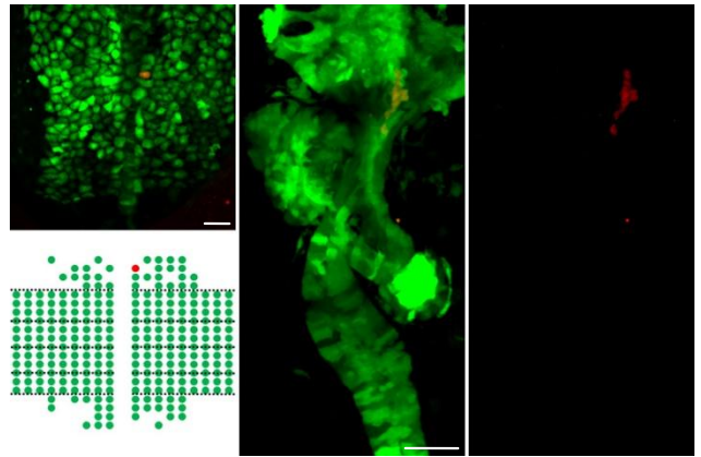
R-A-c1r2 (n=5)
