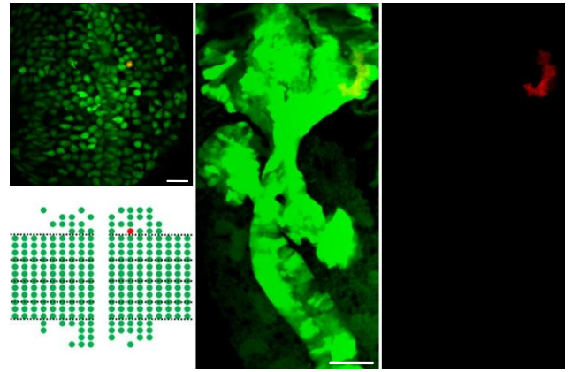
R-A-c3r4 (n=5)
