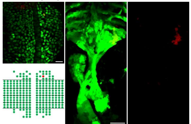
R-A-c3r3 (n=5)
