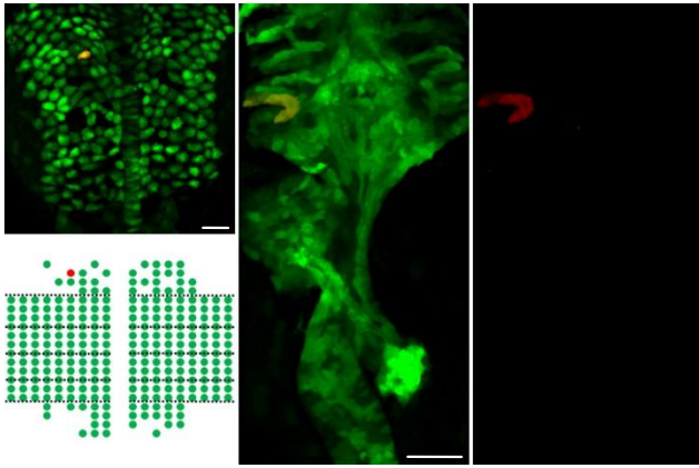
L-A-c4r2 (n=5)
