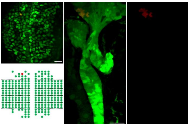
L-A-c3r2 (n=5)
