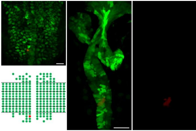
L-P-c1r2 (n=5)
