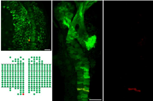
L-P-c1r4 (n=5)
