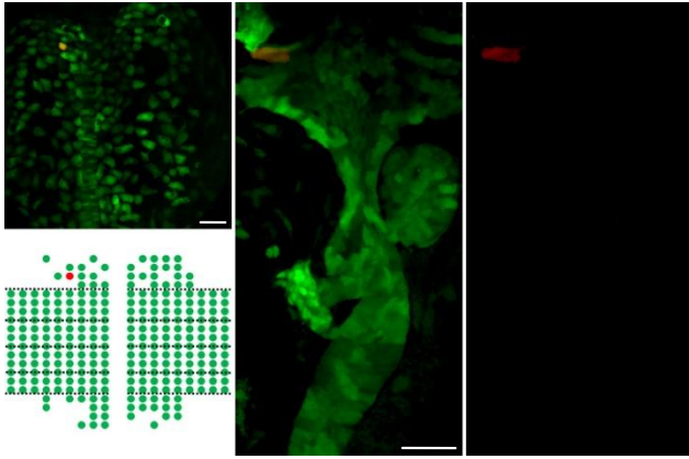
L-A-c4r3 (n=5)
