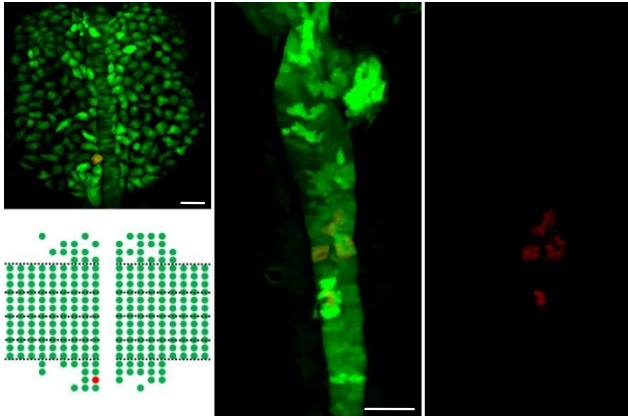
L-P-c1r3 (n=5)
