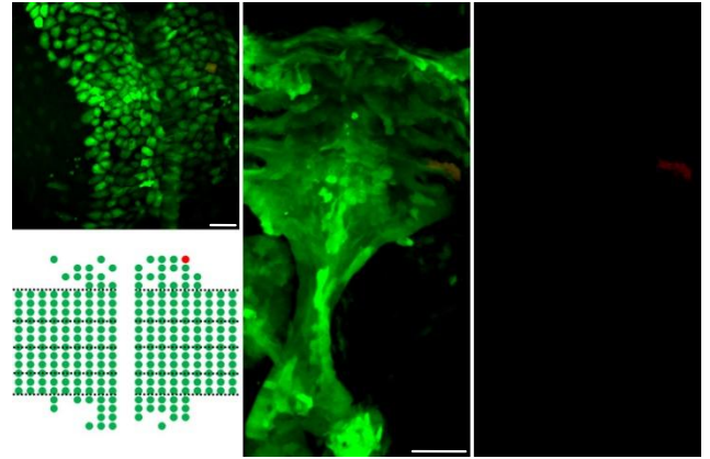
R-A-c5r1 (n=5)
