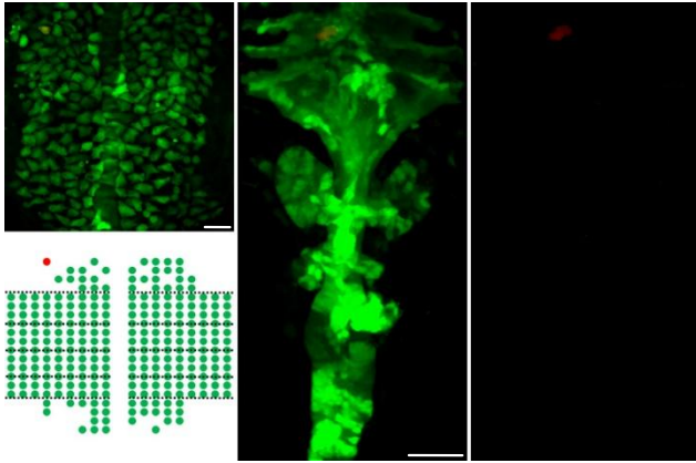
L-A-c6r1 (n=5)
