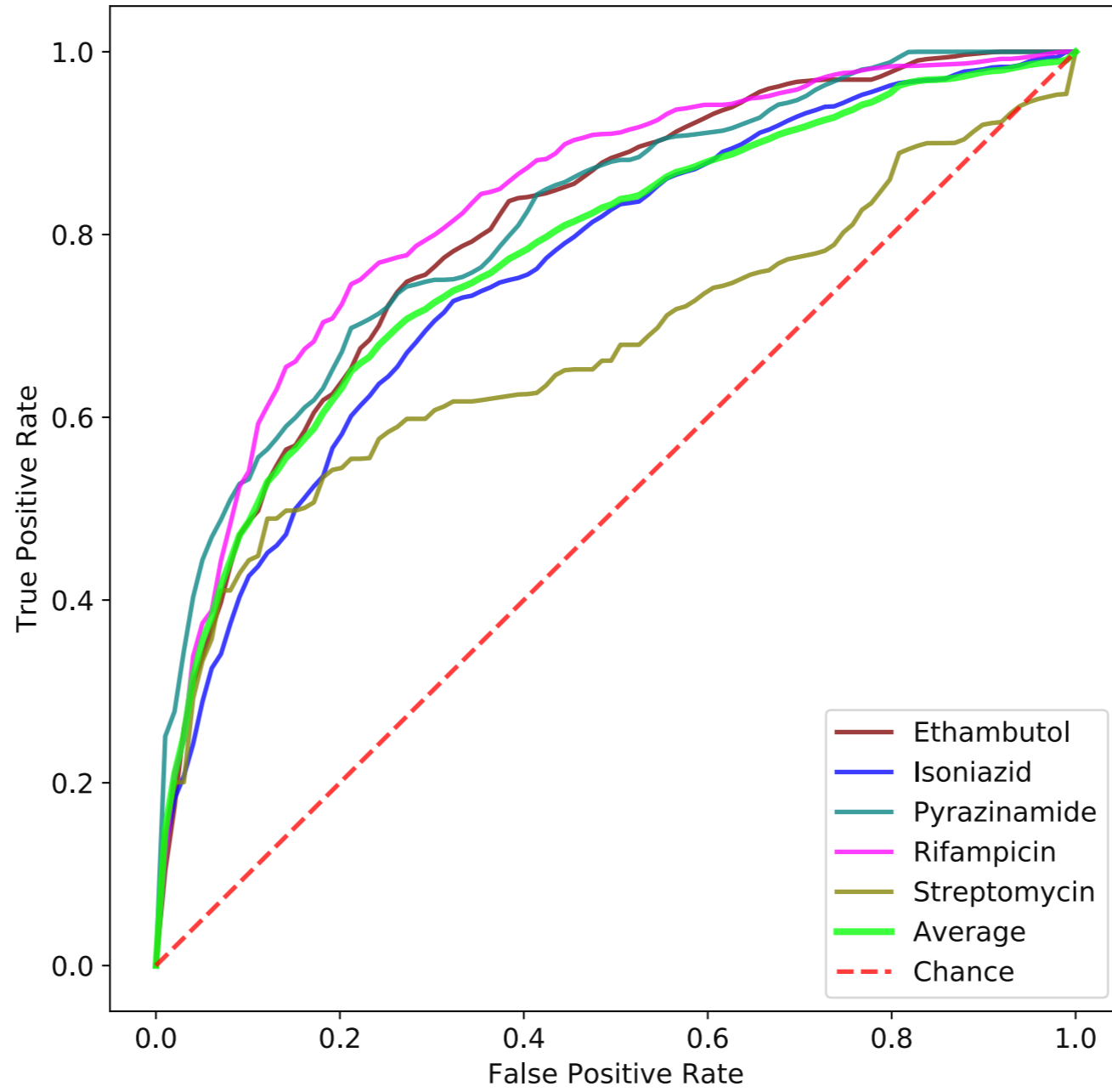
M. tuberculosis
