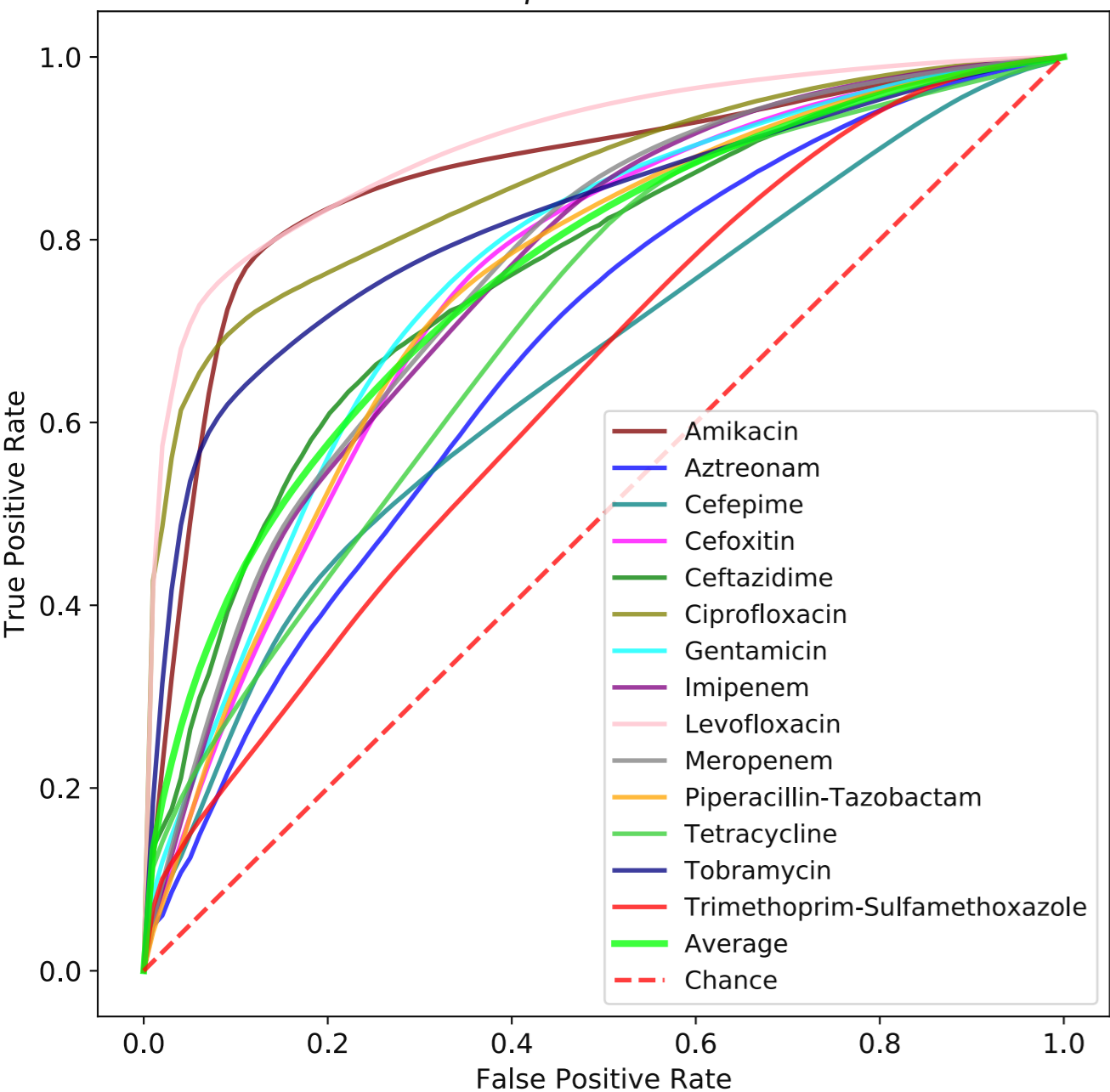
K. pneumoniae
