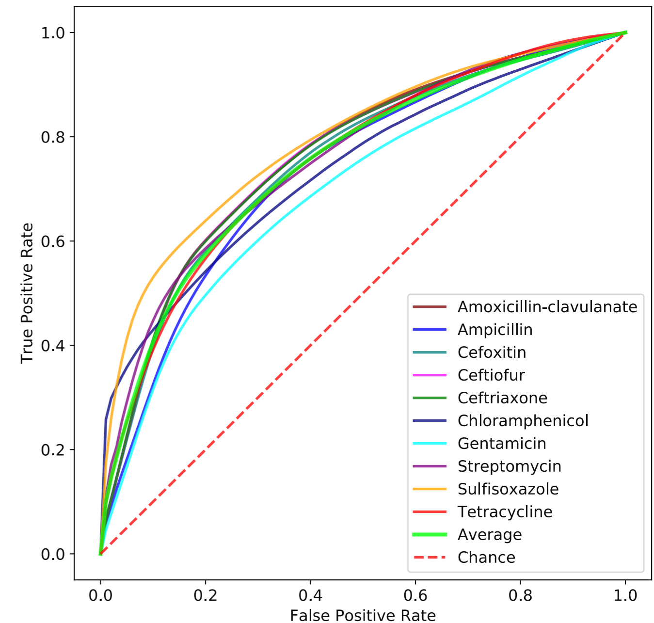
S. enterica
