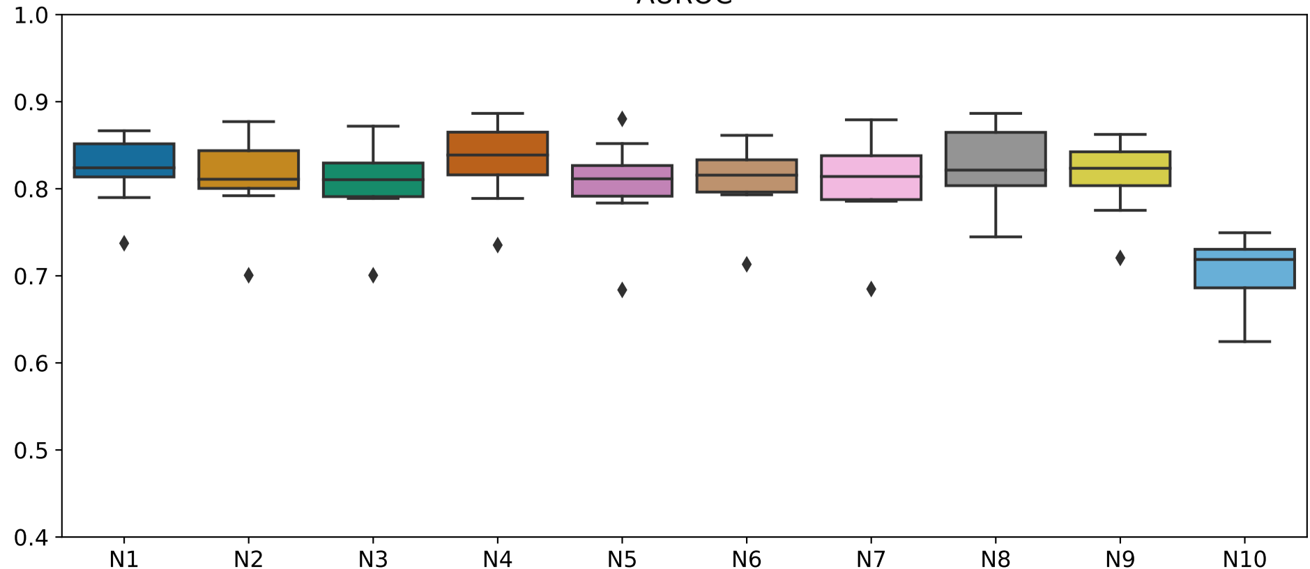
AUROC
