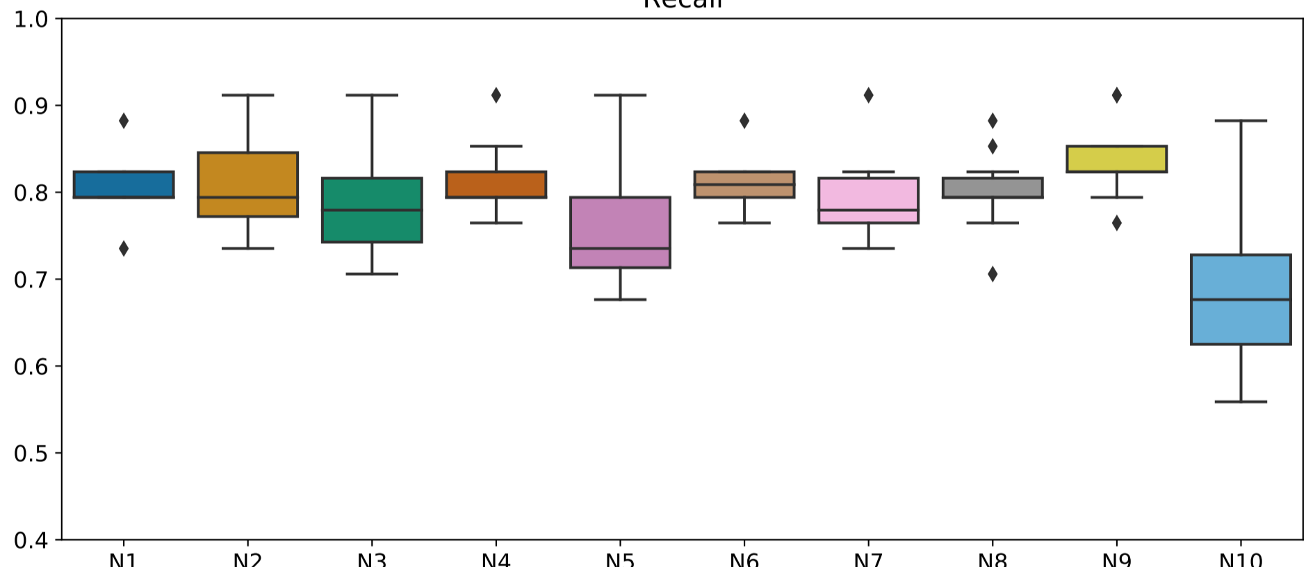
F1 Score
