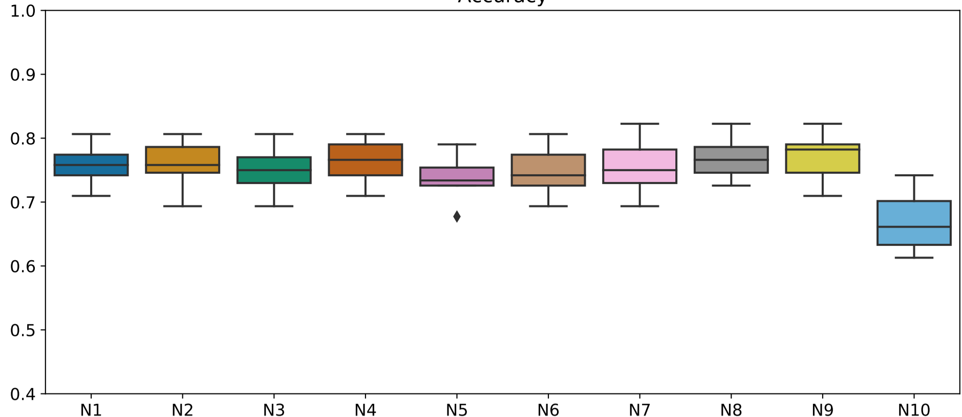
Precision
