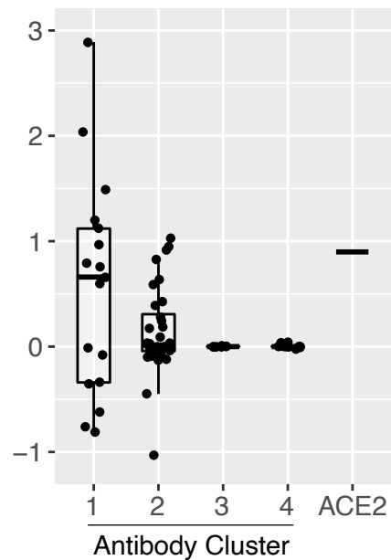
T478K
