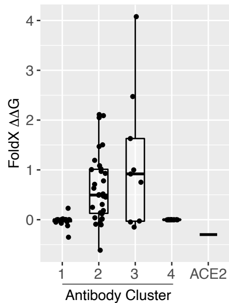
E484Q
