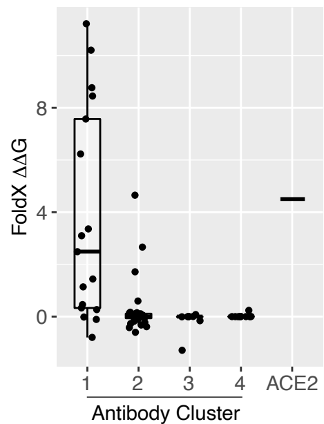
N501Y
