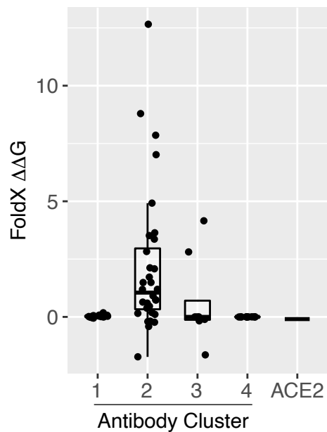
E484K
