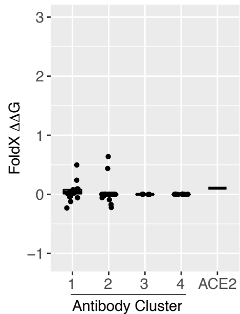
N501Y
