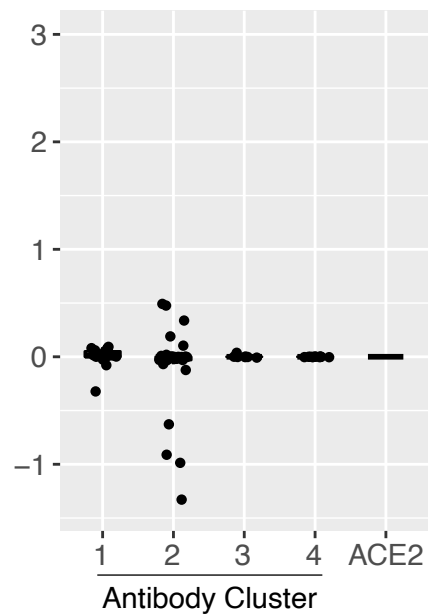
T478K
