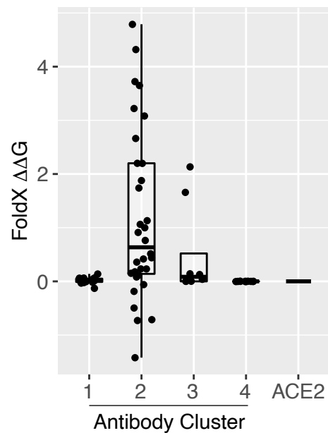
E484Q
