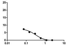
\alpha B.1.1.7/501Y.V1
