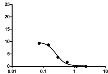
\gamma P.1/501Y.V3
