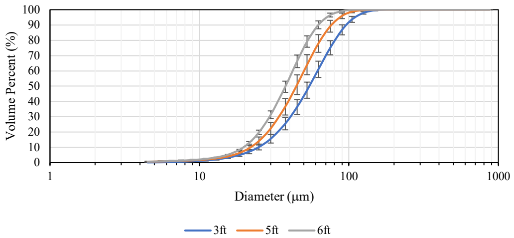
PX300 Red nozzle Cumulative Distribution DI
