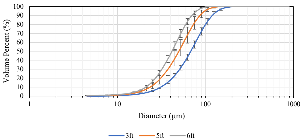
R40 Cumulative Distribution DI
