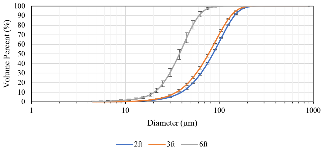
PX200 HH ES Off Cumulative Distribution DI
