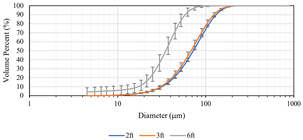
PX200 HH ES On Cumulative Distribution DI
