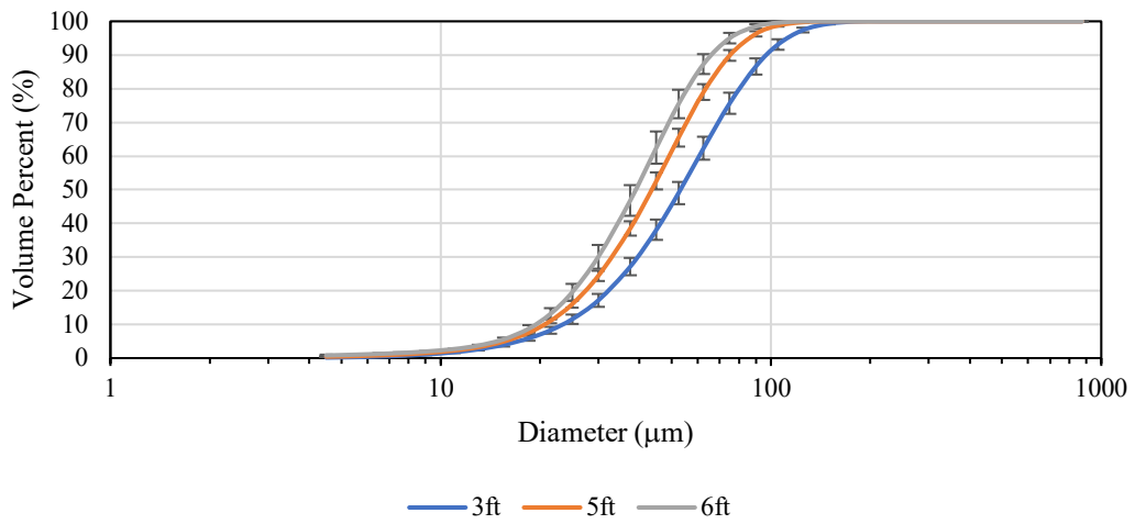
PX300 green nozzle Cumulative Distribution DI
