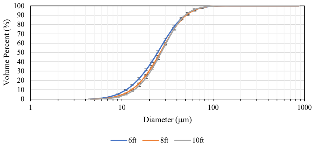
SC-ET Cumulative Distribution DI
