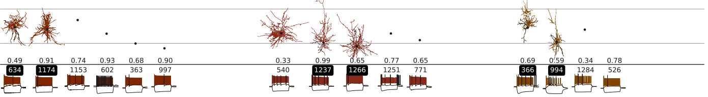
Sst Th_1
