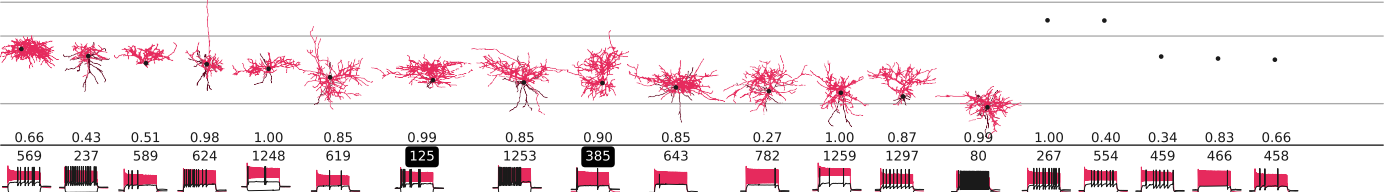
Pvalb Kank4
