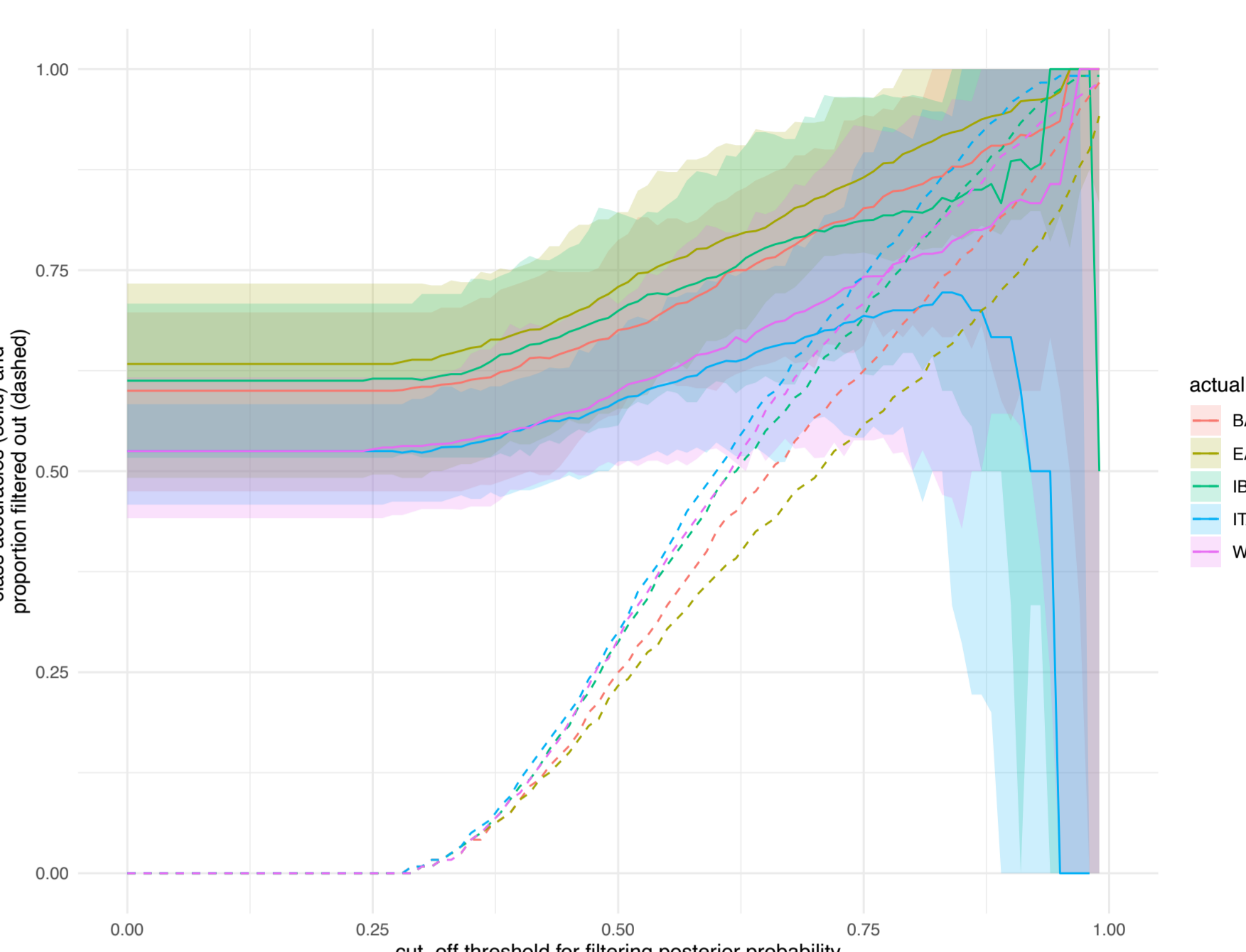
e) SSR5
