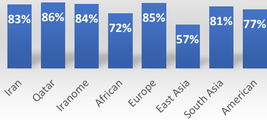
rs3797814-G-A ERAP1
