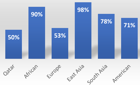
rs4830983 - ACE2
