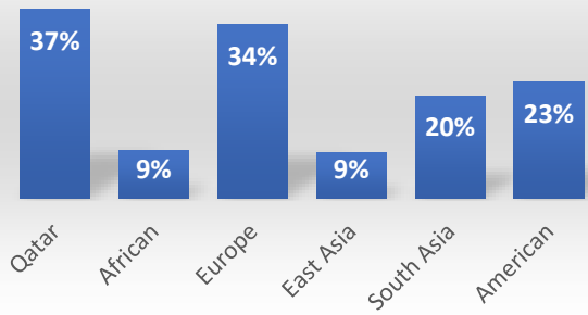
rs3797814-G-A ERAP1
