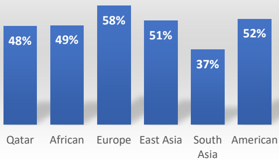
rs9264255-T-A HLA-B
