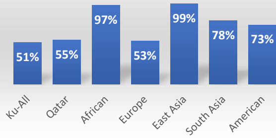
rs5936011 - ACE2
