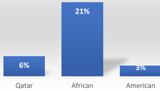
rs5936029 - ACE2
