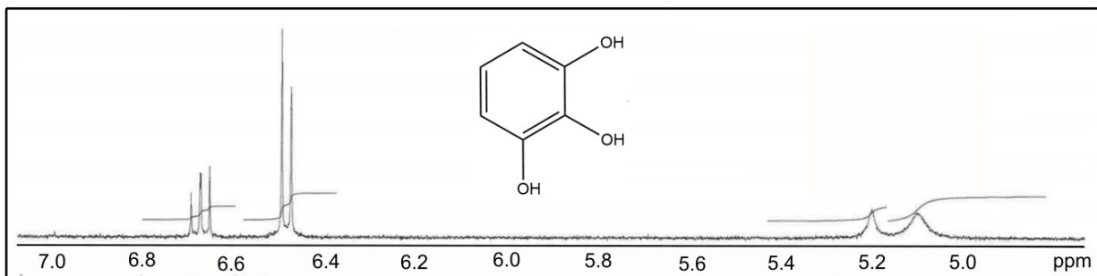
Figure S9. 1 H-NMR of standard 1,2,3-benzenetriol (pyrogallol).
