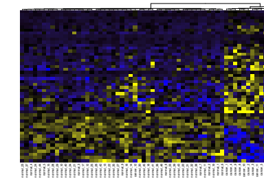
100 DMRs
