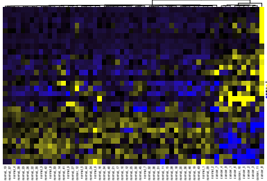
30 DMRs
