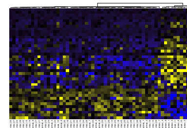
50 DMRs
