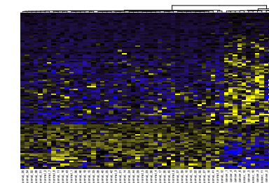
100 DMRs
