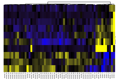
20 DMRs
