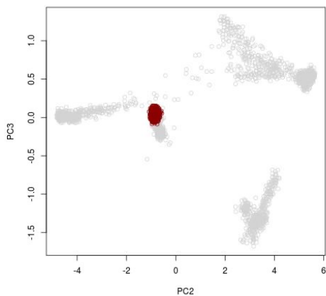
(B) PC2 vs PC3
