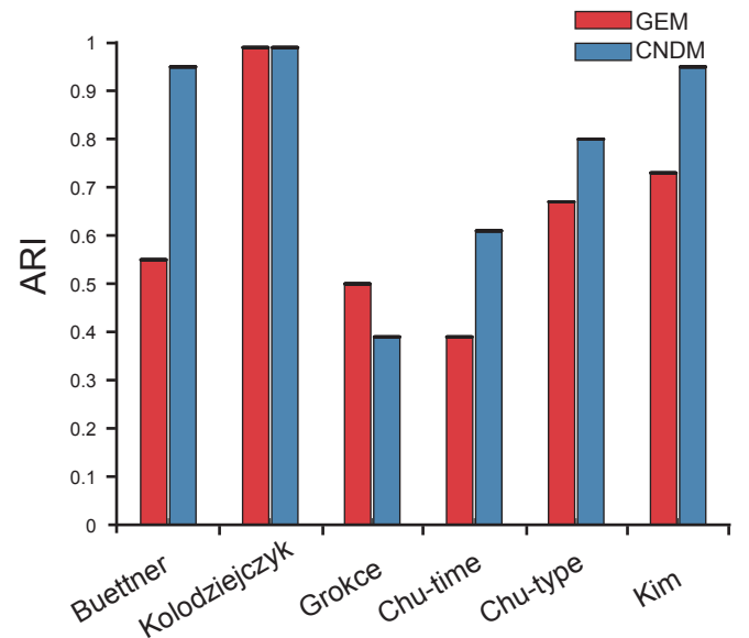
t-SNE + Hierarchical
