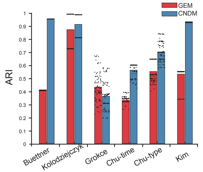
t-SNE + Hierarchical
