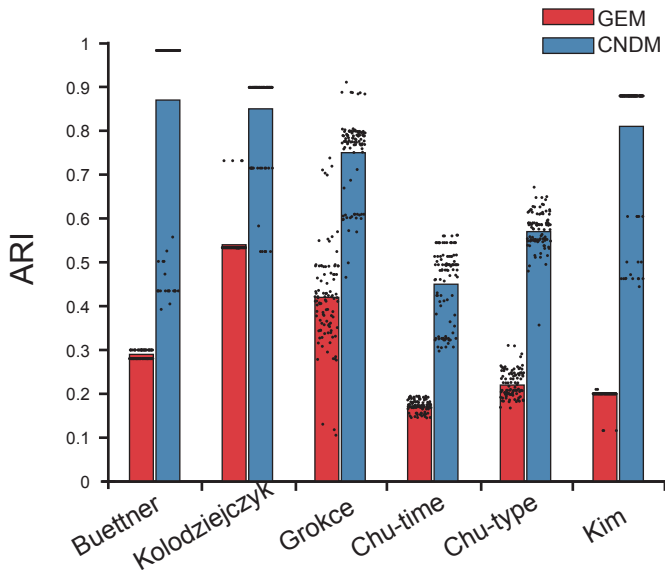
Hierarchical
