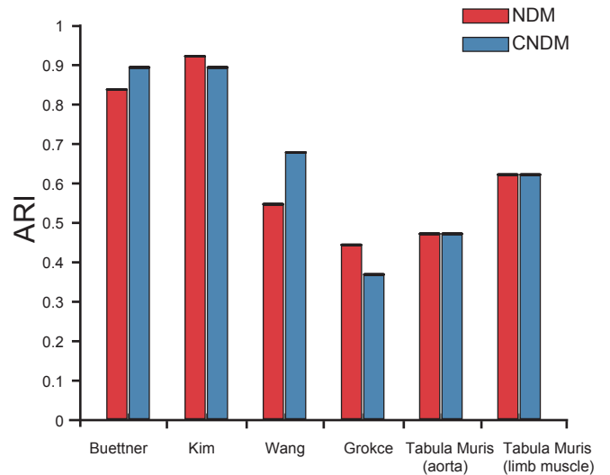
t-SNE + Hierarchical
