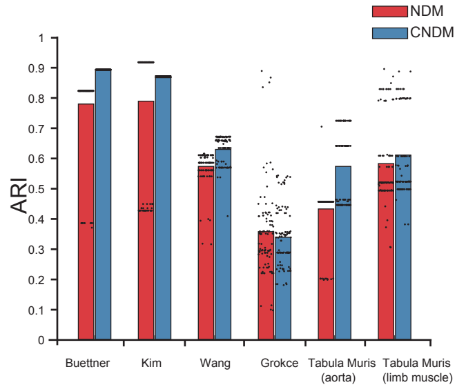
t-SNE + K-means
