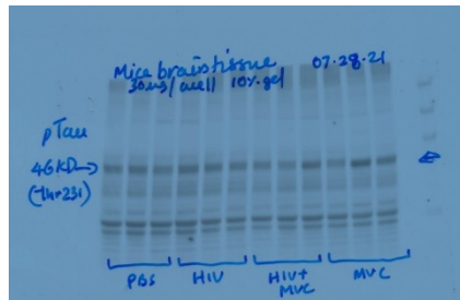
pTau (Thr231)
