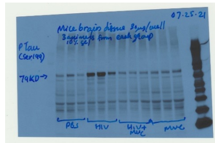
pTau (Ser199)
