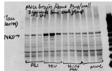
pTau (Ser199)
