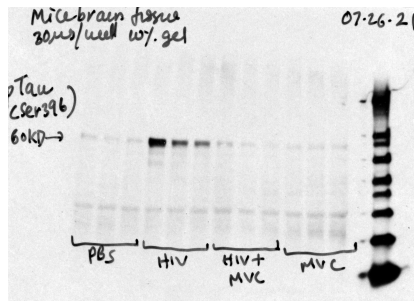
pTau (Ser396)
