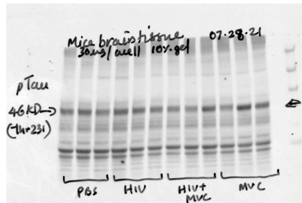
pTau (Thr231)
