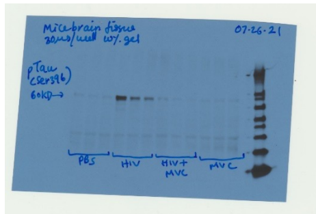
pTau (Thr231)
