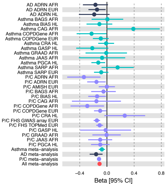
chr12q13.3 rs1059513
