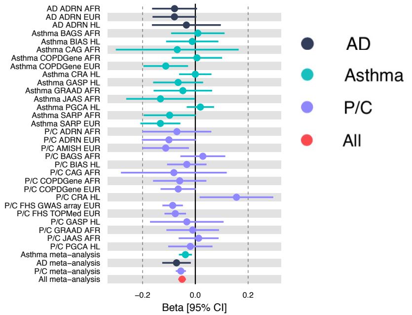
chr11q13.5 rs7936323
