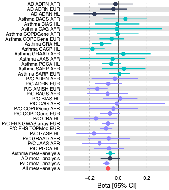
chr12q13.3 rs1059513
