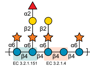
Xyloglucan
