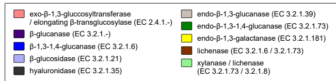
Cellulose
