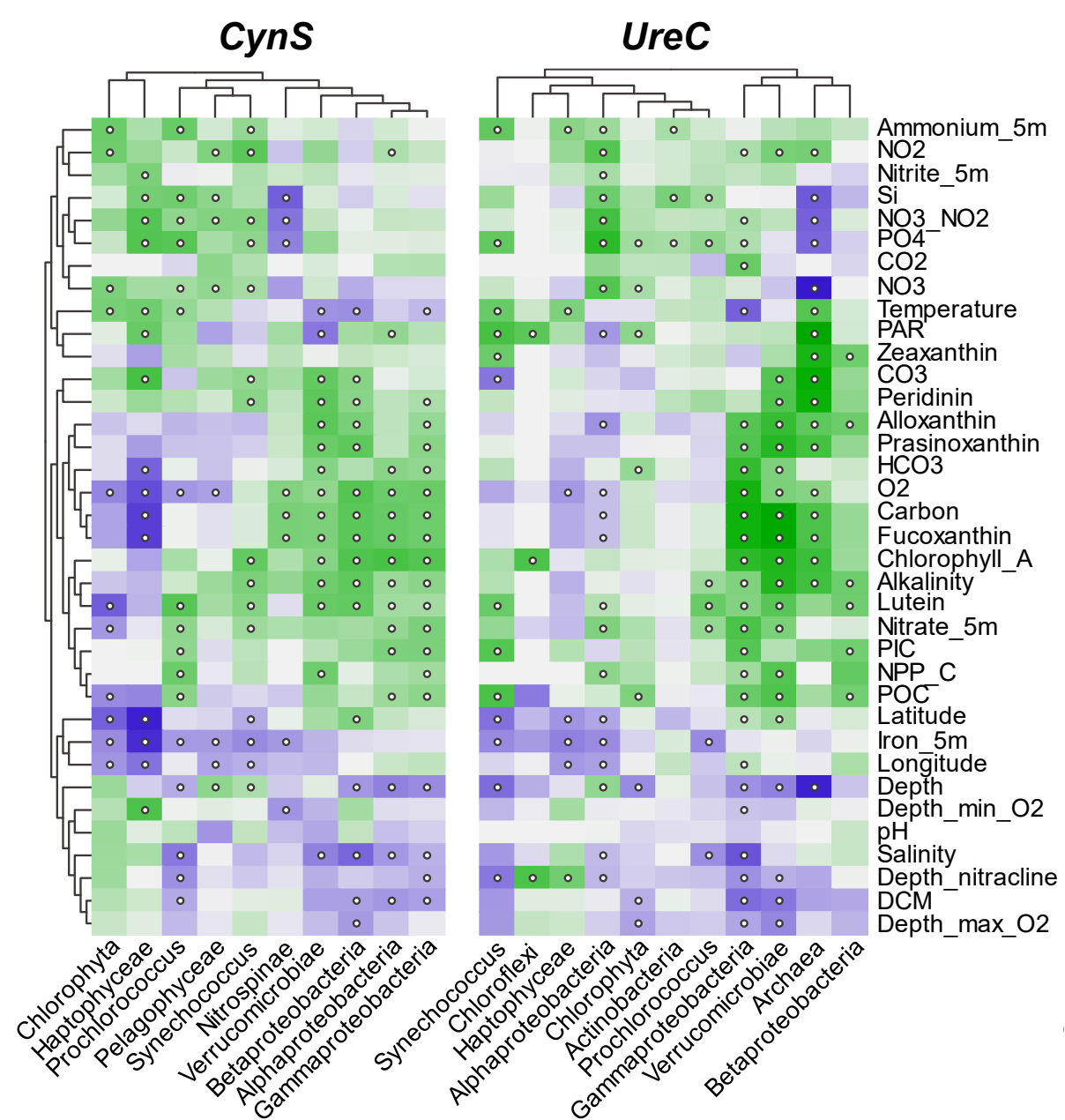
(d) Gene Abundance (0.22-3 \mu\text{m} fraction)
