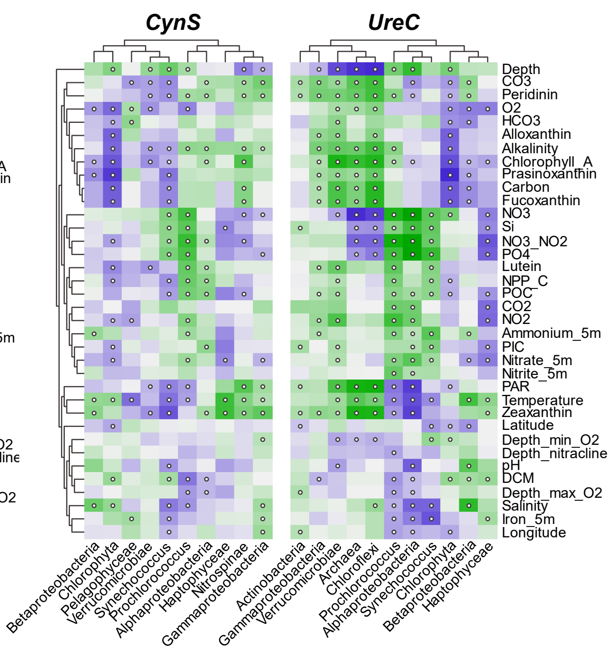
(d) Gene Abundance (0.22-3 \mu\text{m} fraction)
