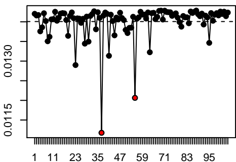
tau2.del
