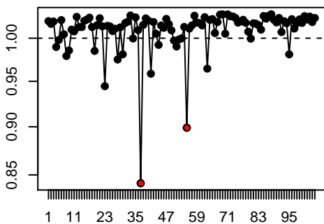
cov.r
