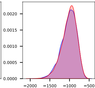
Posterior density
