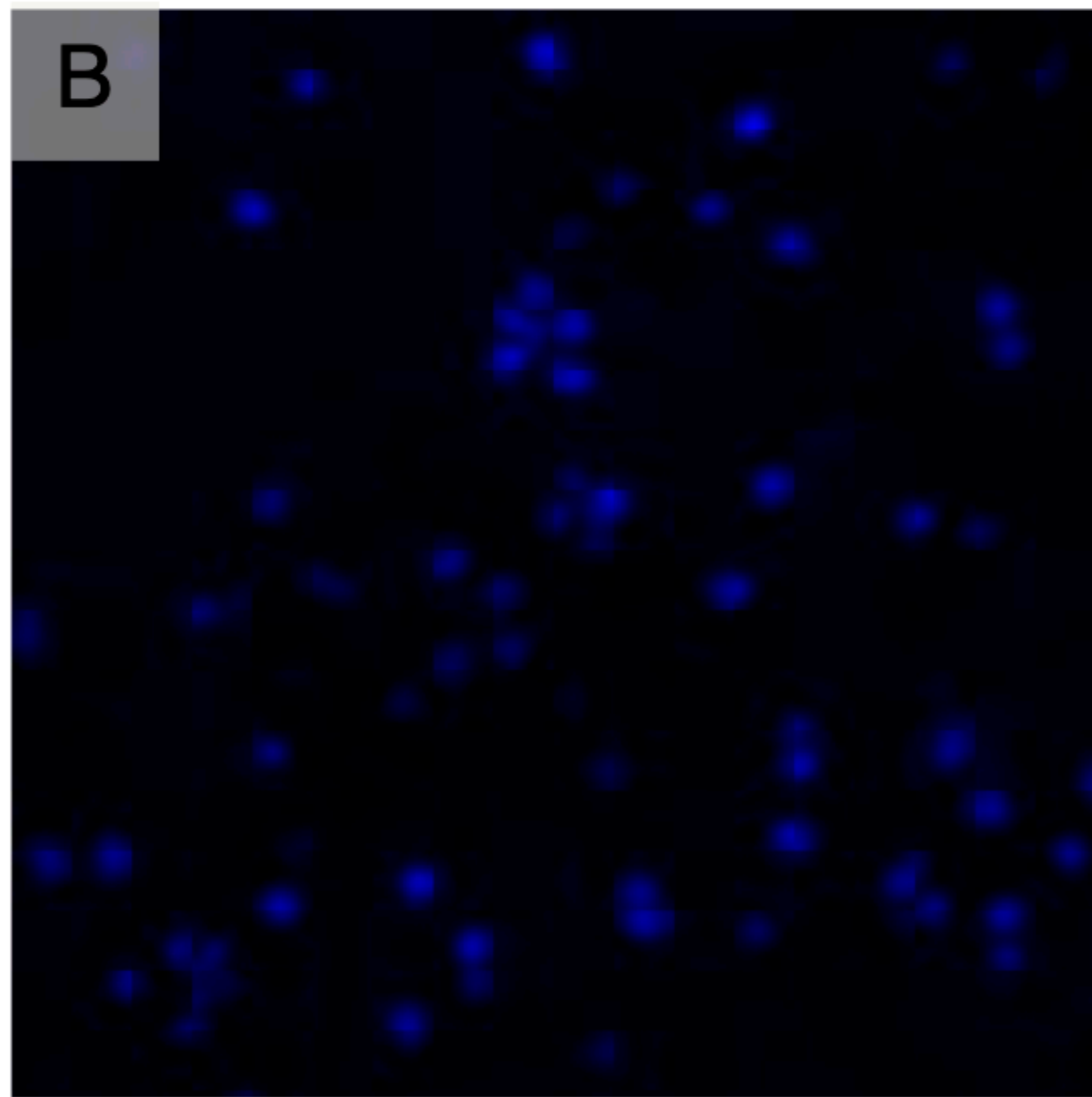
Eub338-II & III (Verrucomicrobia-Planctomycetes)
