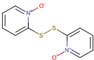
DIPYRITHIONE
