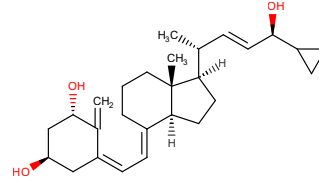
CALCIPOTRIENE
