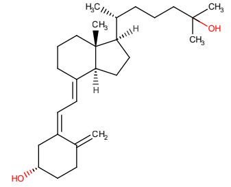
INECALCITOL
