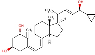
CALCIPOTRIOL
