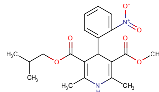
NISOLDIPINE
