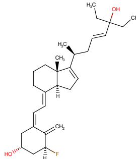
ELOCALCITOL
