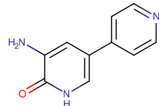
INAMRINONE
