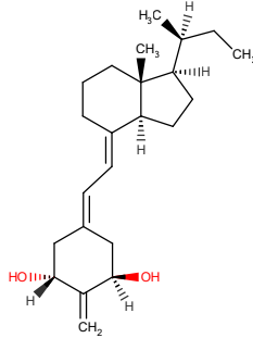
ELOCALCITOL
