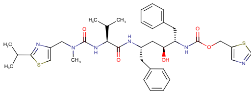
RITONAVIR
