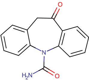
TEMEFOS
