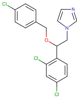
RITONAVIR
