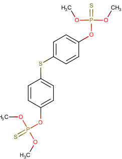
TEMEFOS
