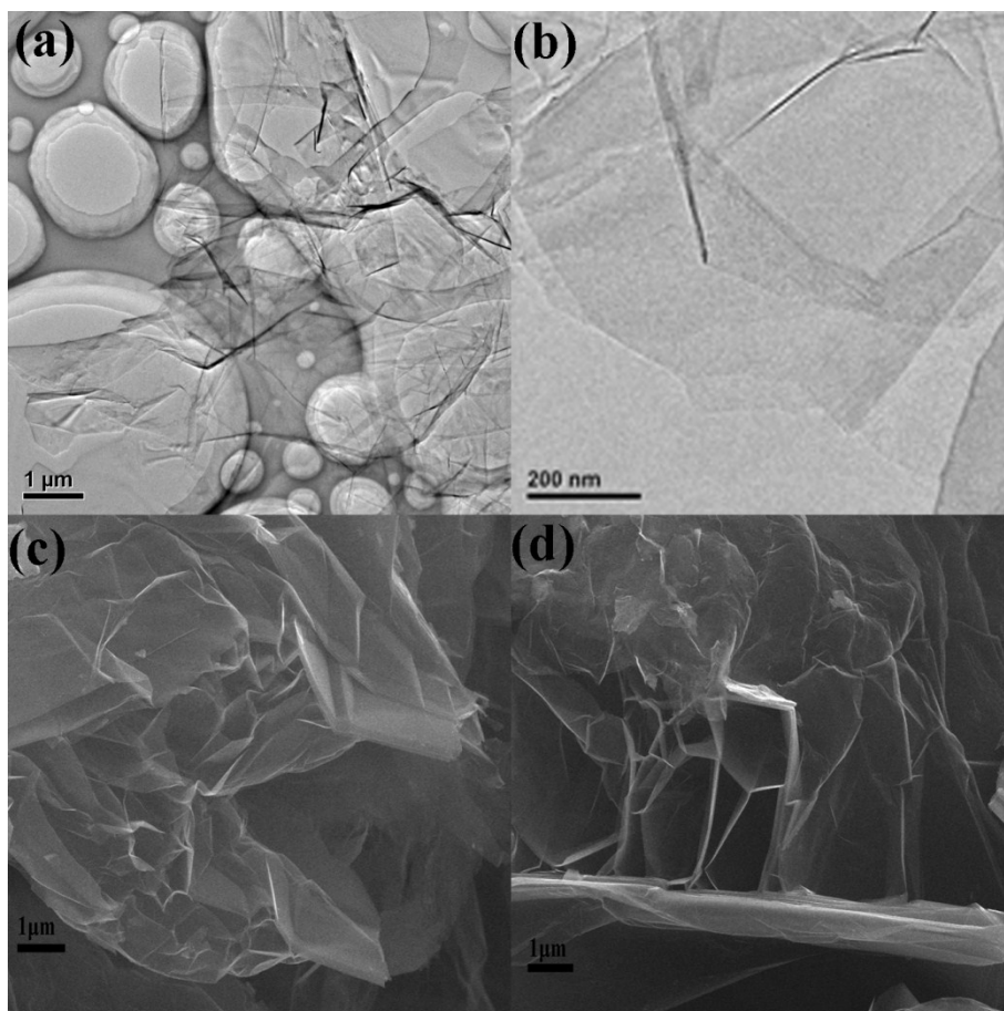
Fig. S1. (a, b) TEM images of HG300. (c, d) SEM images of HG300.
