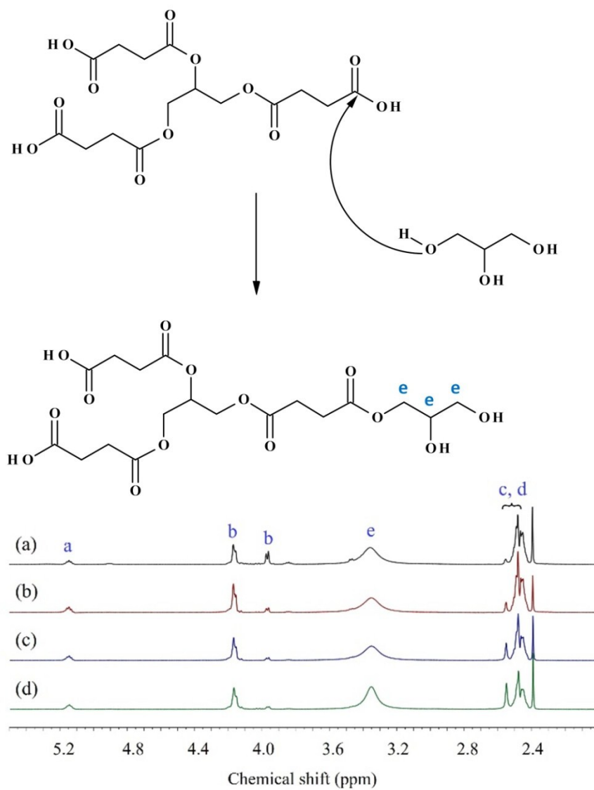
Fig. S2 ^1\text{H} NMR spectra of (a) Gly-SA90, (b) Gly-SA110, (c) Gly-SA130 and (d) Gly-SA150.
