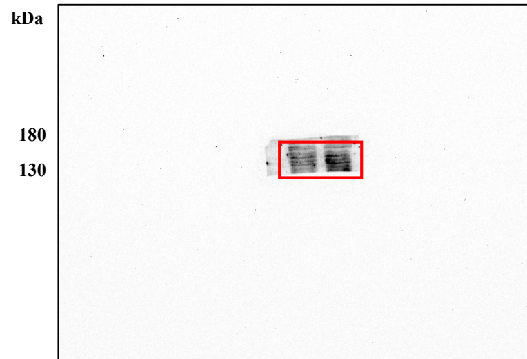
Anti-p-ASK1(Thr845)
