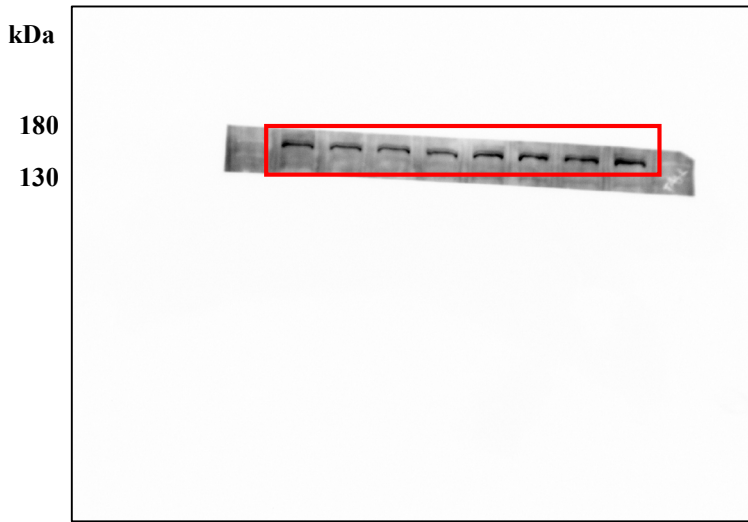
Anti-p-ASK1(Thr845)
