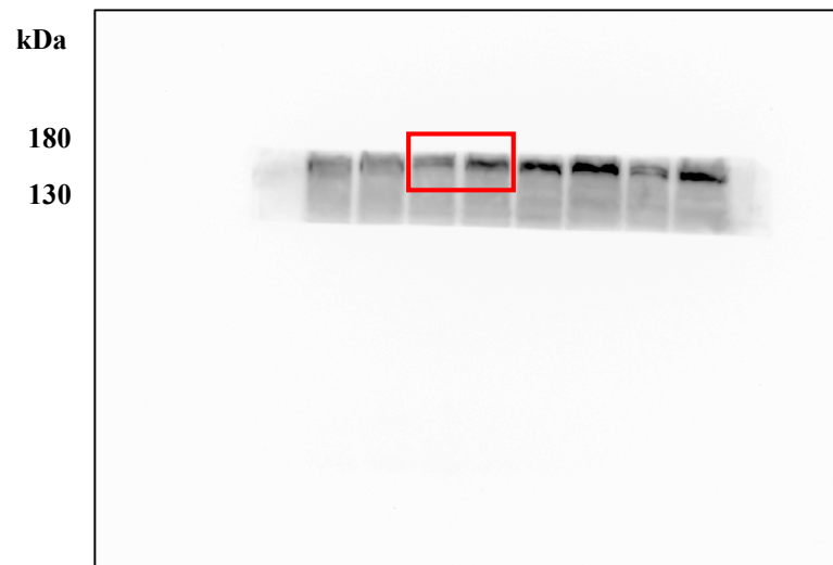
Anti-p-ASK1(Thr845)
