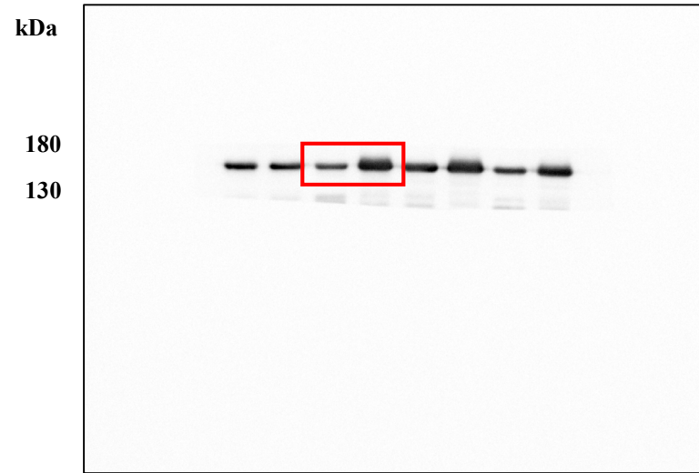
HCT116 Anti-p-ASK1(Thr845)
