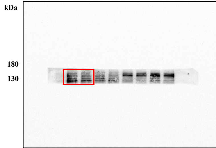
Anti-p-ASK1(Thr845)
