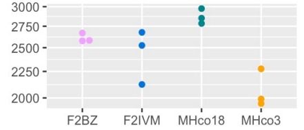
HCON_00098130:pgp-1
