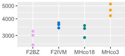
HCON_00004450:pgp-2
