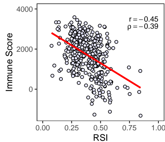
HGG
