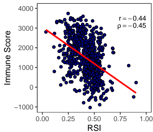
LUAD
