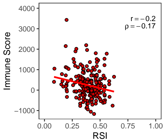
PRAD
