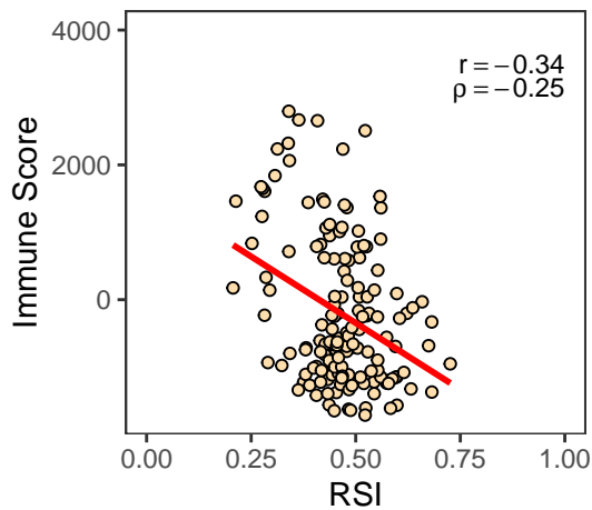
NE
