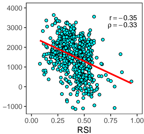
OVCA
