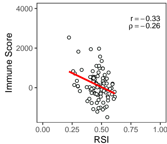
STAD
