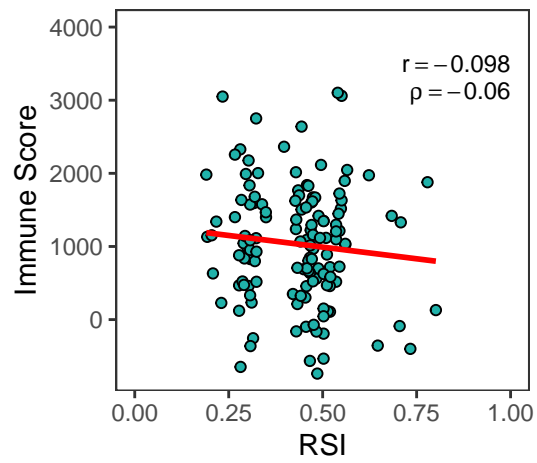
ESCA
