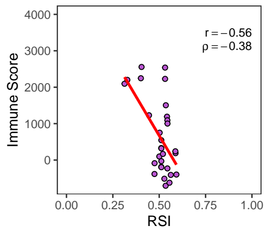
MELA
