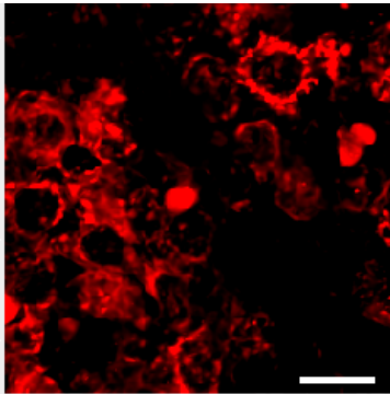
FITC
