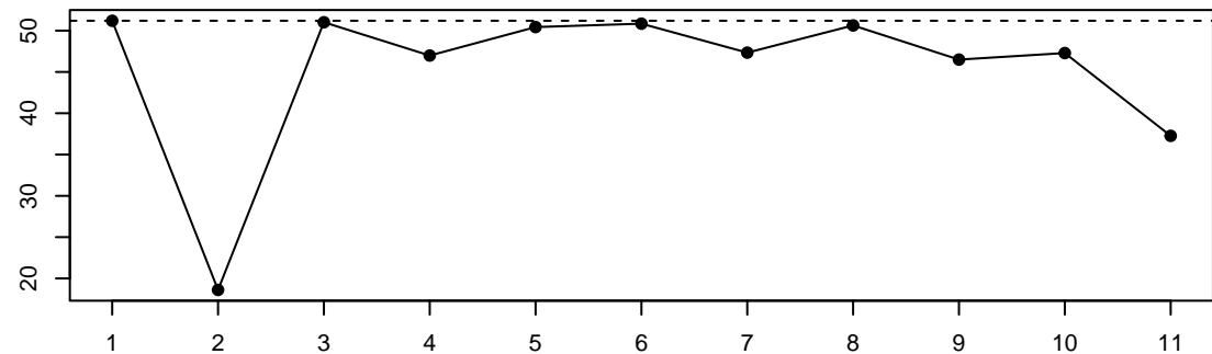
QE.del
