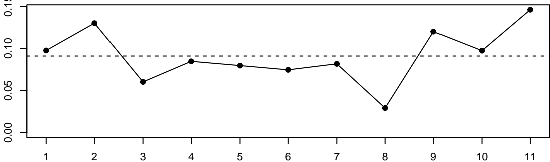
hat
