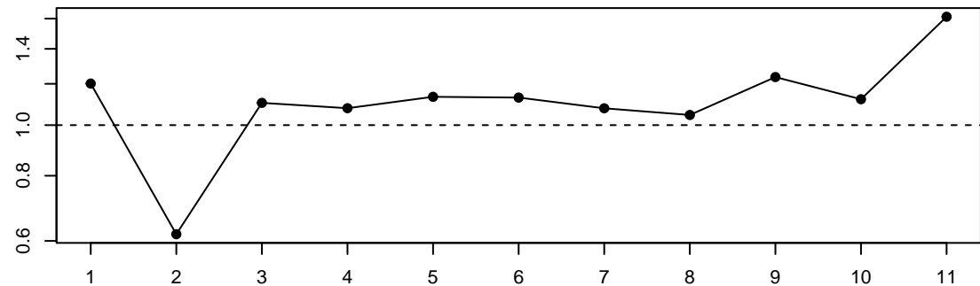
cov.r
