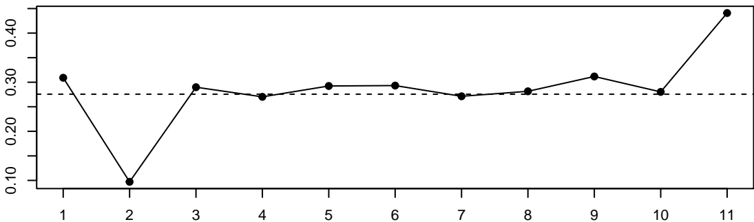
tau2.del
