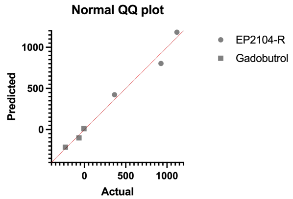
E2.2. Q-Q plot
