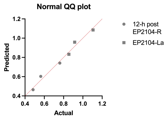
E2.4. Q-Q plot
