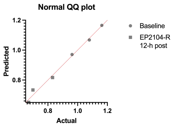
E2.3. Q-Q plot
