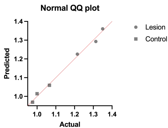
E2.11. Q-Q plot
