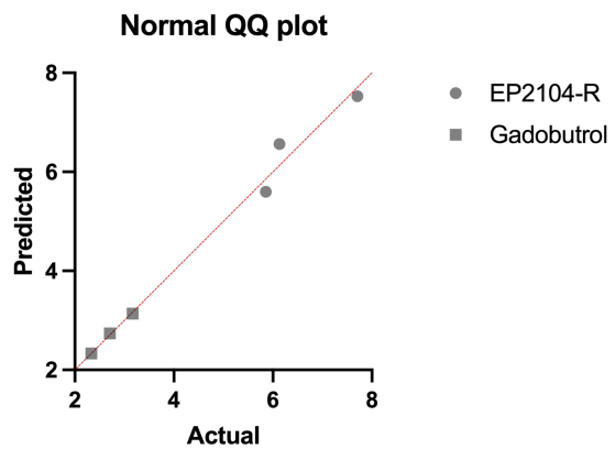
E2.10. Q-Q plot
