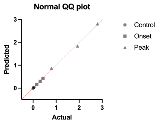
E2.7. Q-Q plot
