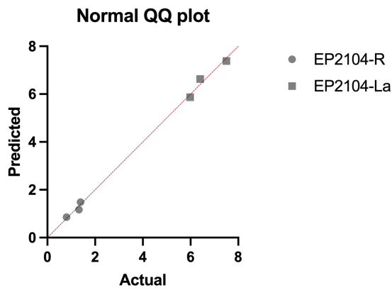
E2.5. Q-Q plot
