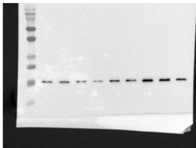
Tom20 (ab186734)
