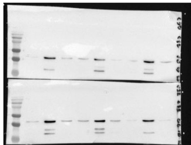
Mcl-1
