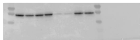
Bax
