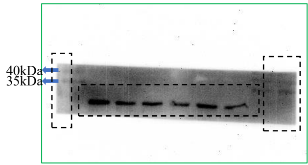
LAMP1 100KDa
