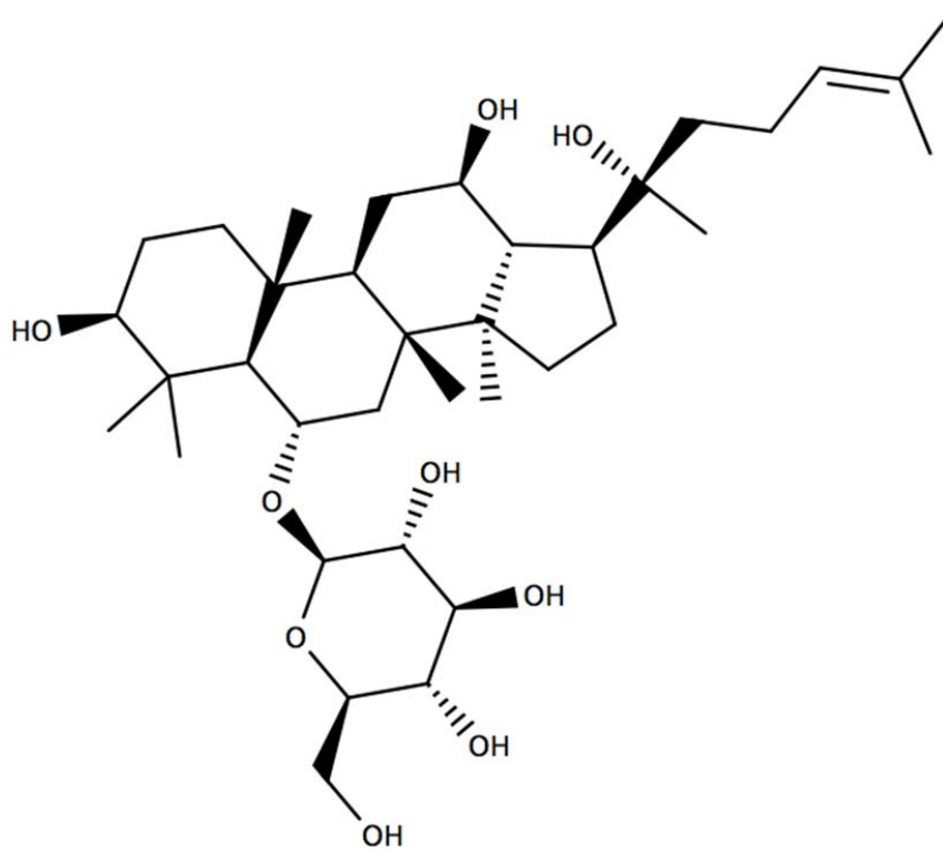
SFigure 1k. 20(S)-Ginsenoside Rh1.
