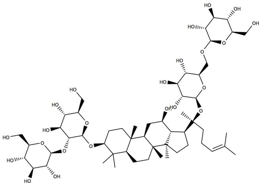
SFigure 1a. Ginsenoside Rb1.
