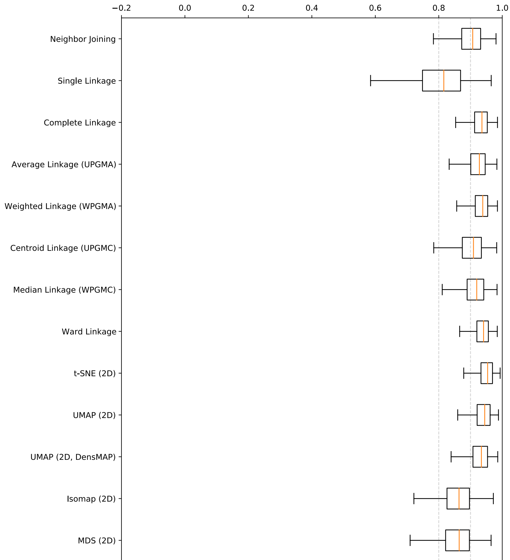
Trustworthiness (k=10)
