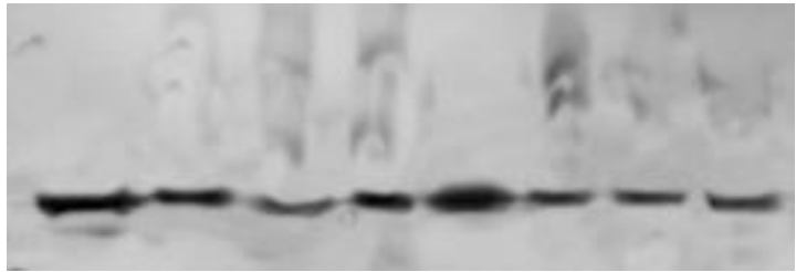
190 kD CD206
