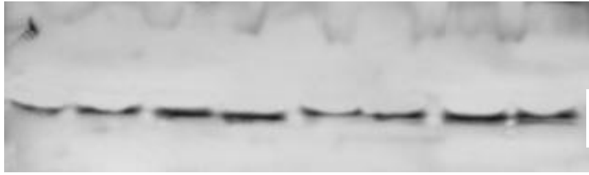
60-85 kD CD86
