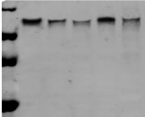
130-180 kD P-gp
